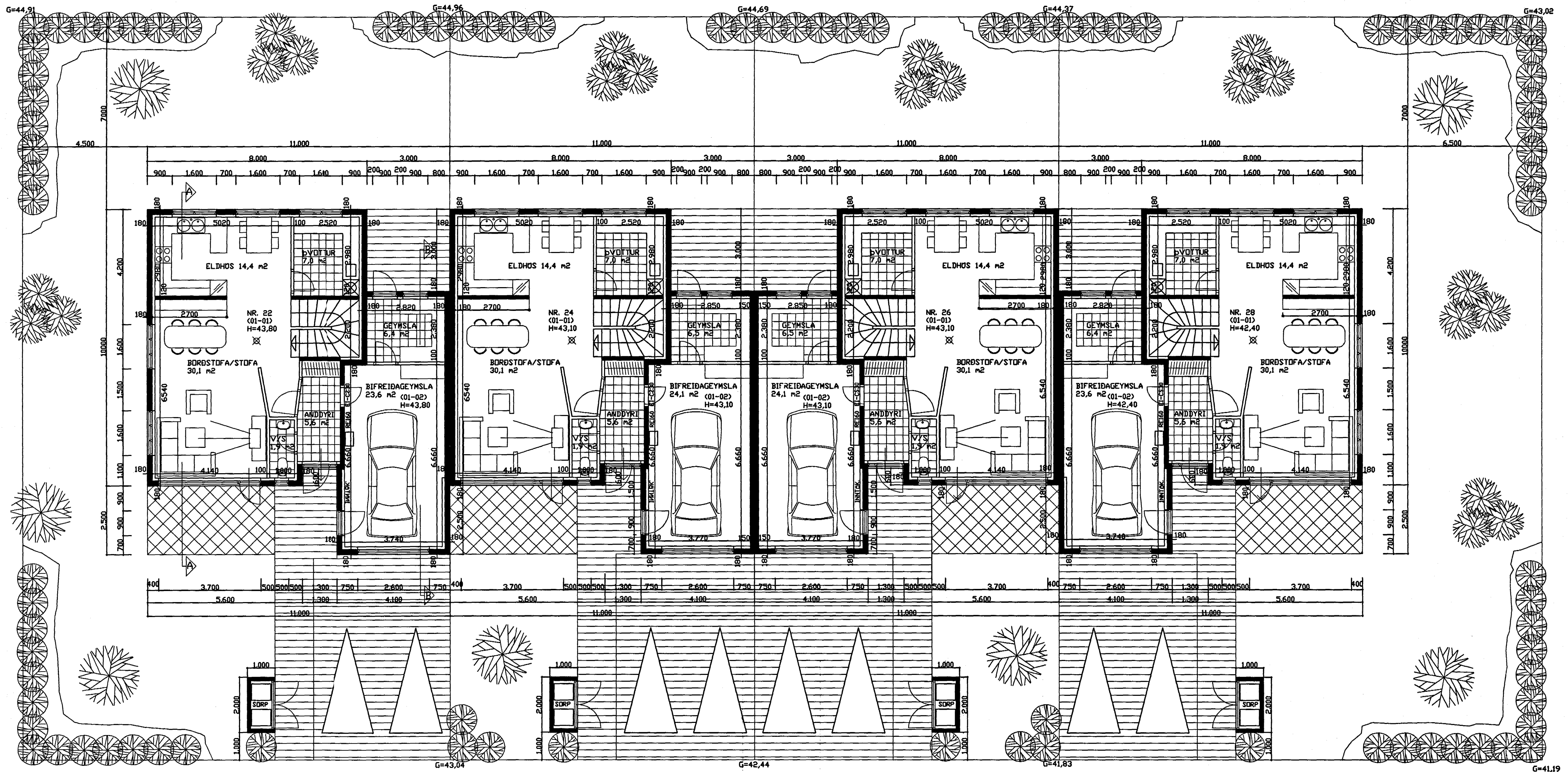
GRUNNMYND 1 HÆÐ MKV. 1:100.
