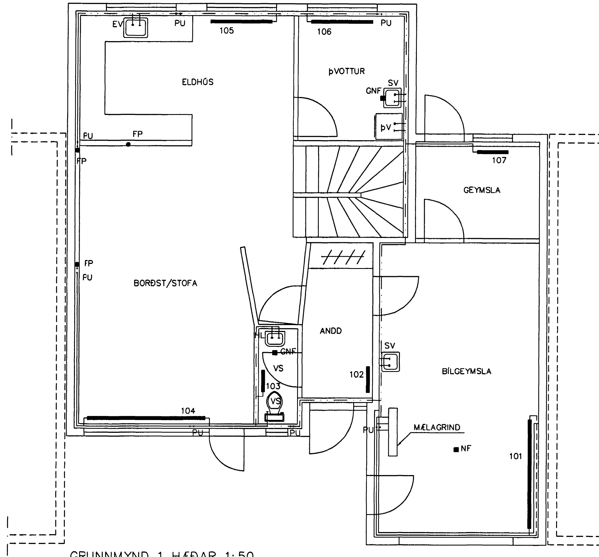
GRUNNMYND 1 HÆÐAR 1:50
