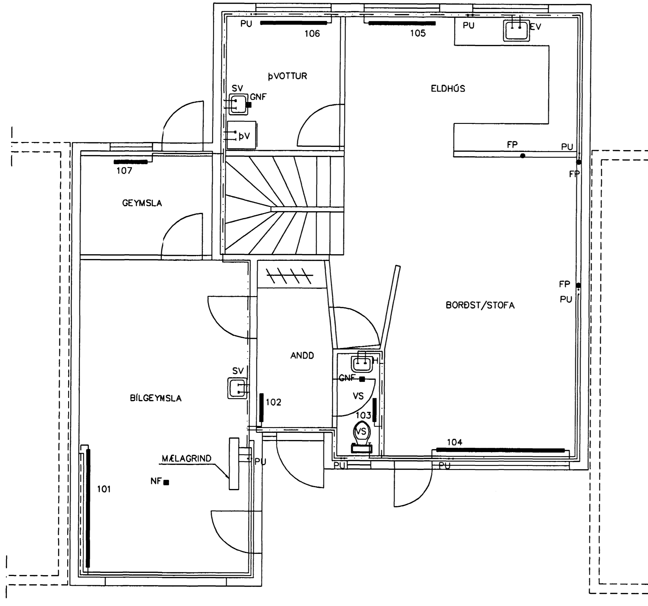
GRUNNMYND 1:50
