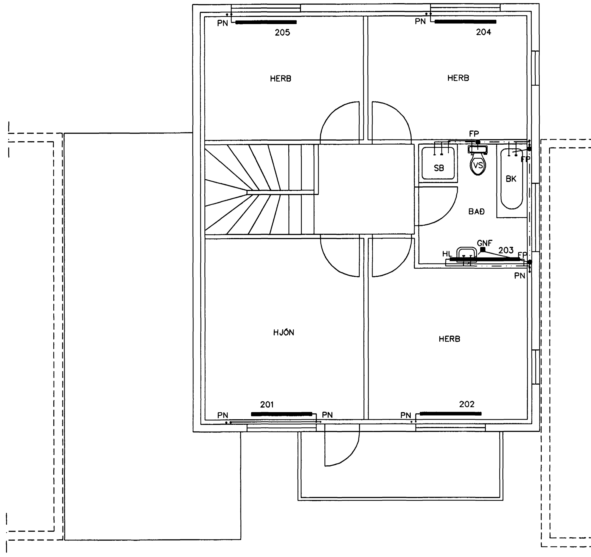
GRUNNMYND 2 HÆÐAR 1:50
