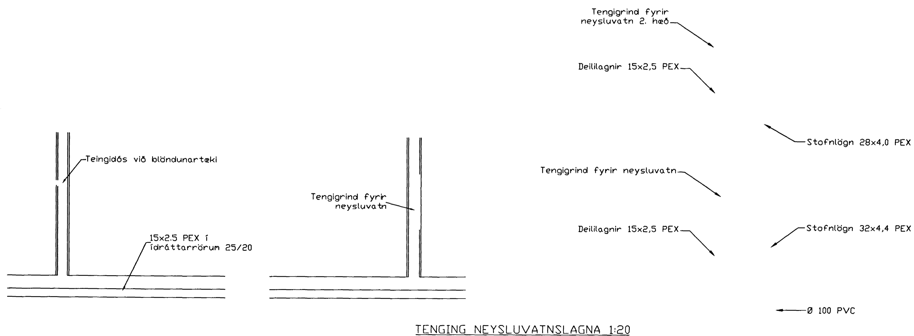
TENGING NEYSLUVATNSLAGNA 1:20
