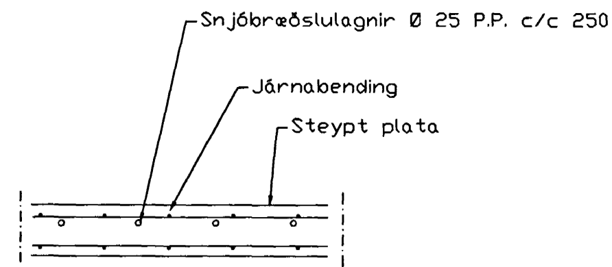
Snjóbræðsla snið, 1:10
