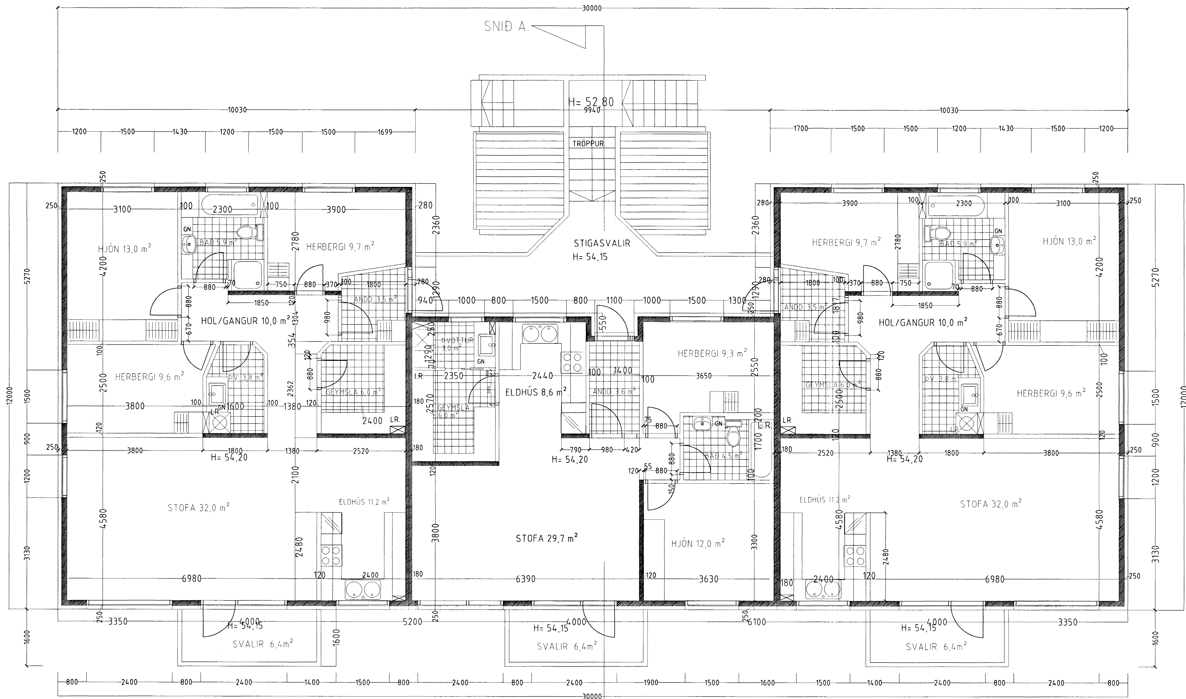
Grunnmynd 2. hæð. mkv. 1:50.
