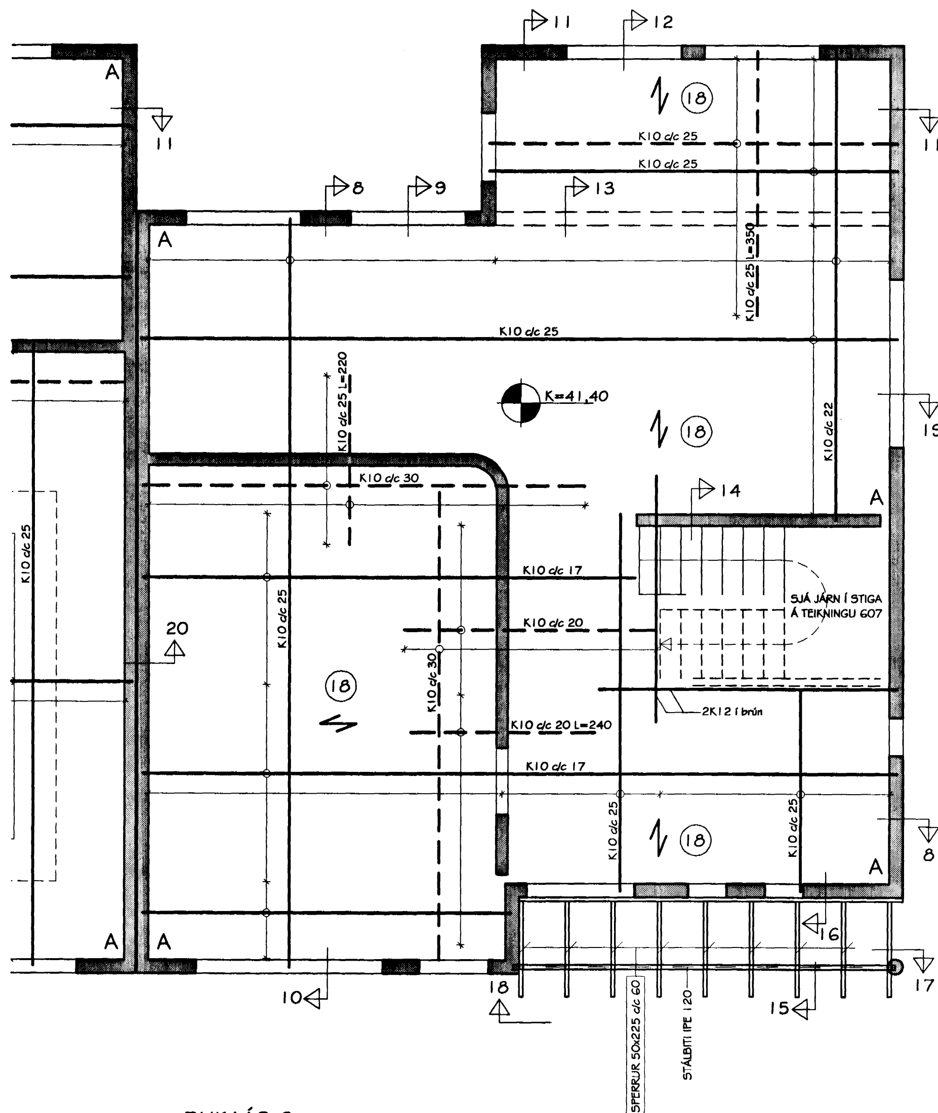
BLIKAÁS 2 JÄRN Í PLÖTU YFIR NEÐRI HÆÐ GRUNNMYND MKV. 1:50
