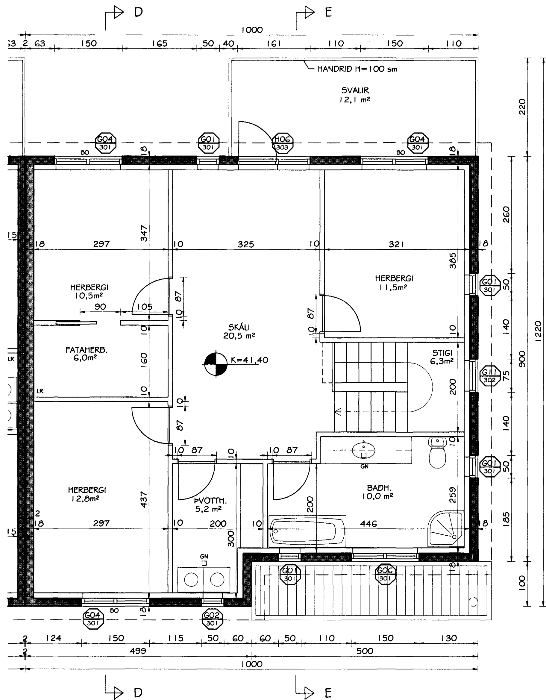
GRUNNMYND EFRI HÆÐAR (HÚS NR. 2) MKV. 1:50
