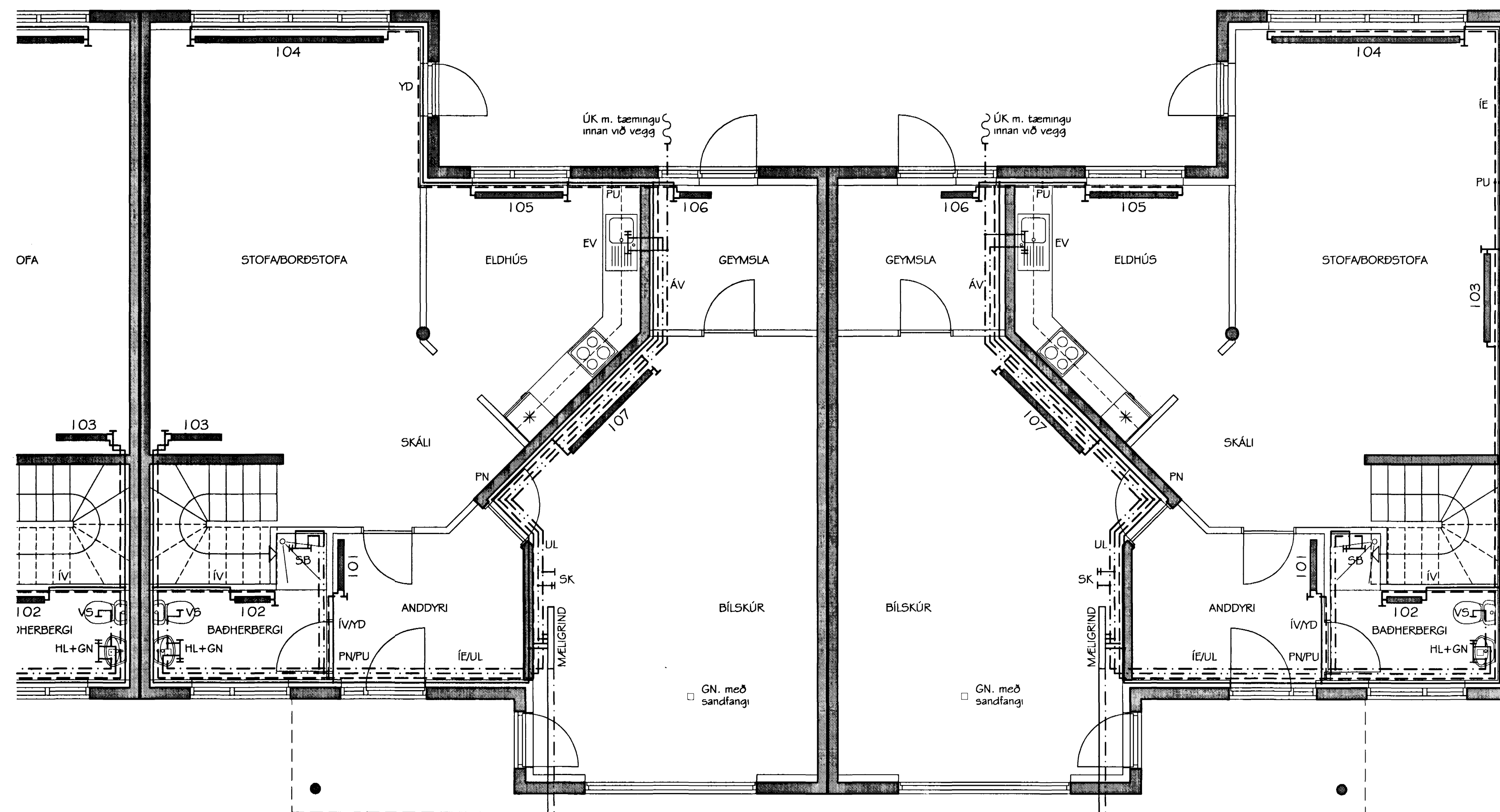
BLIKAÁS 30 OG 32 HITA- OG NEYSLUVATNSLAGNIR GRUNNMYND NEDRI HÆÐAR MKV. 1:50
