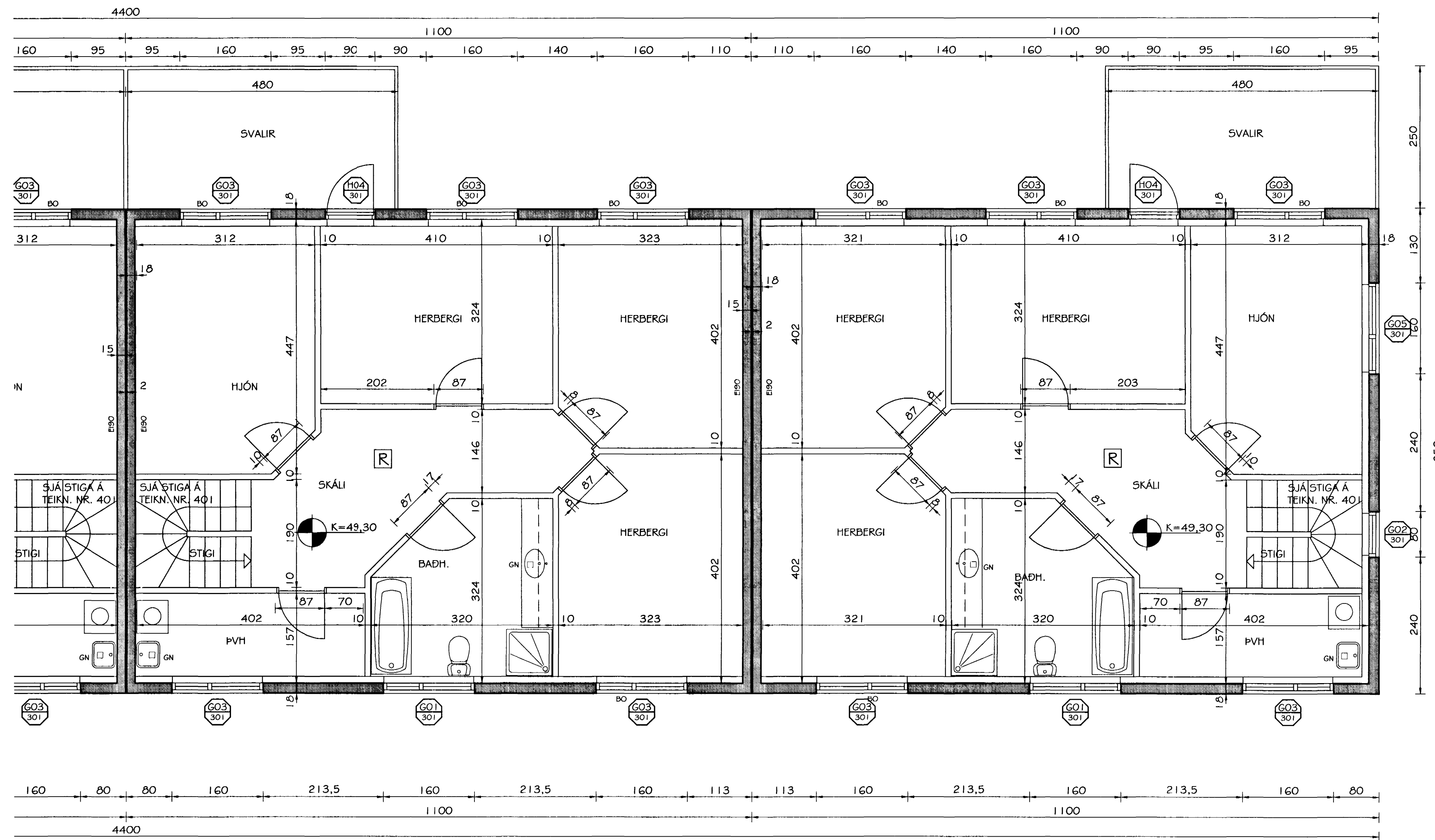
BLIKAÁS 30 OG 32 GRUNNMYND EFRI HÆÐAR MKV. 1:50
