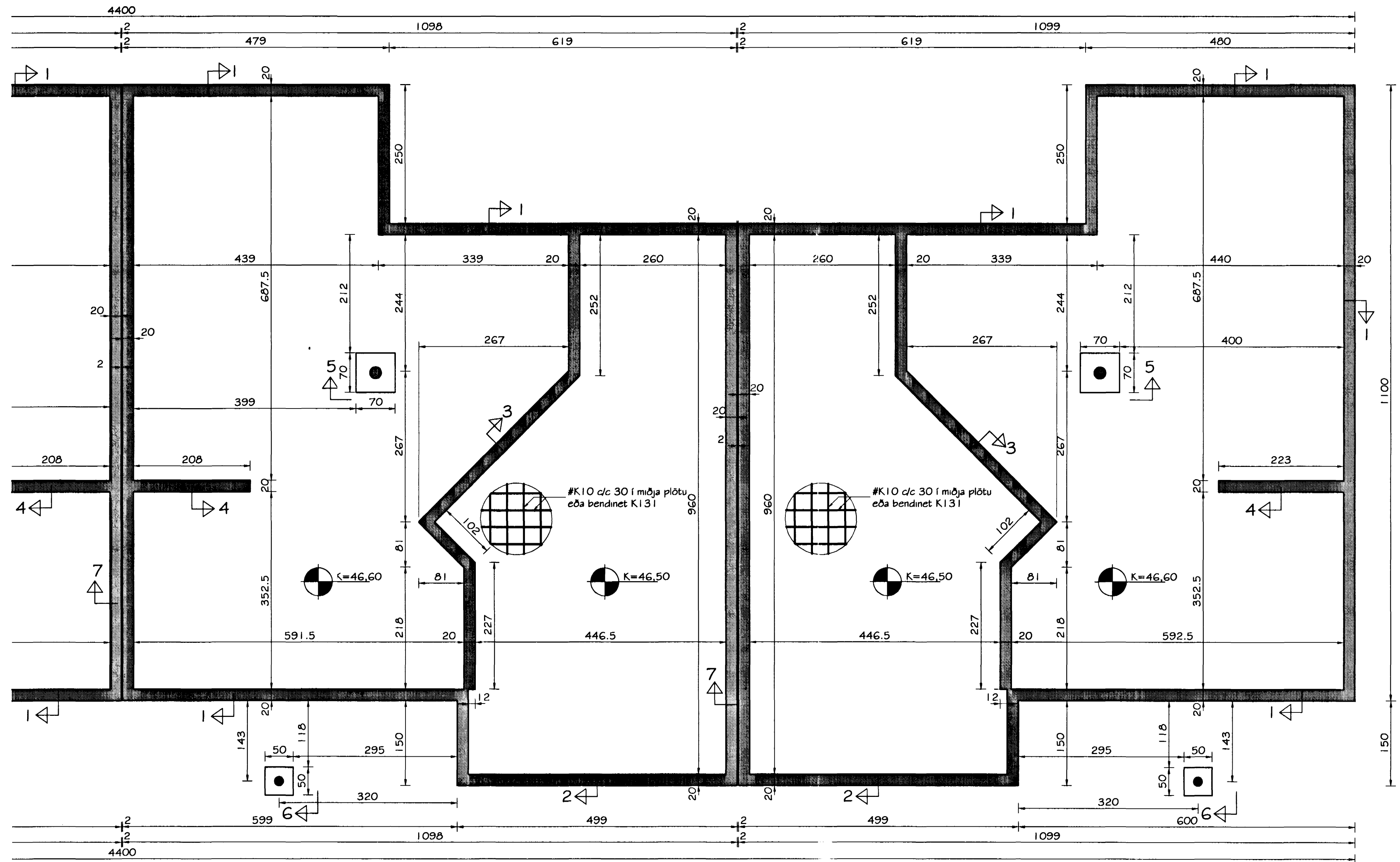
BLIKAÁS 30 OG 32 GRUNNMYND SÖKKLA MKV. 1:50
