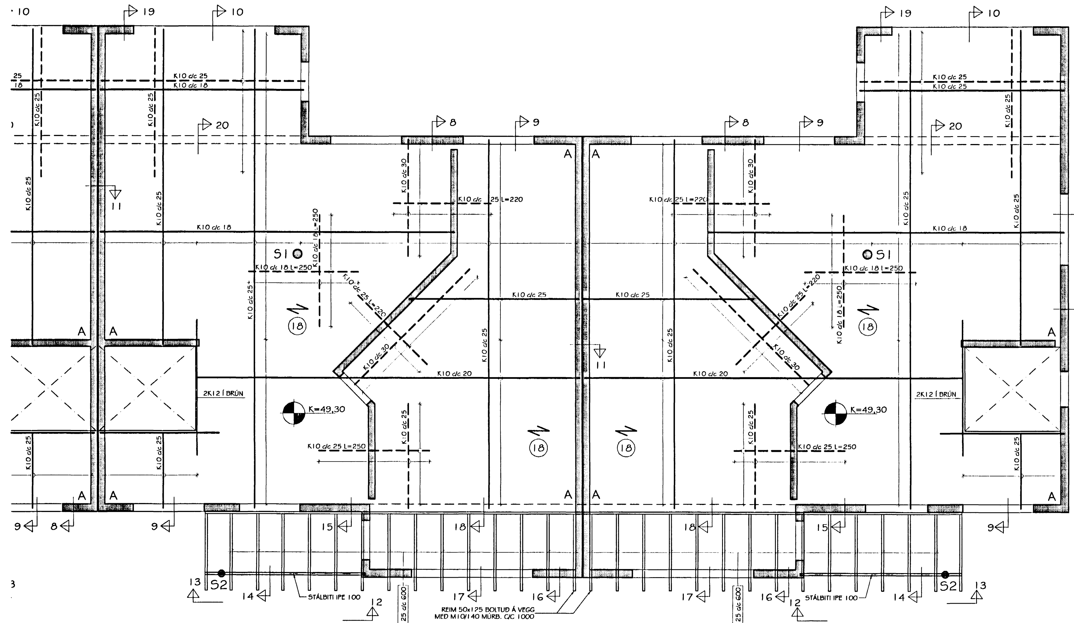
BLIKAÁS 30 OG 32 JÁRN Í PLÖTU YFIR 1. HÆÐ OG GRUNNMÝND PAKVIÐA MKV. 1:50
