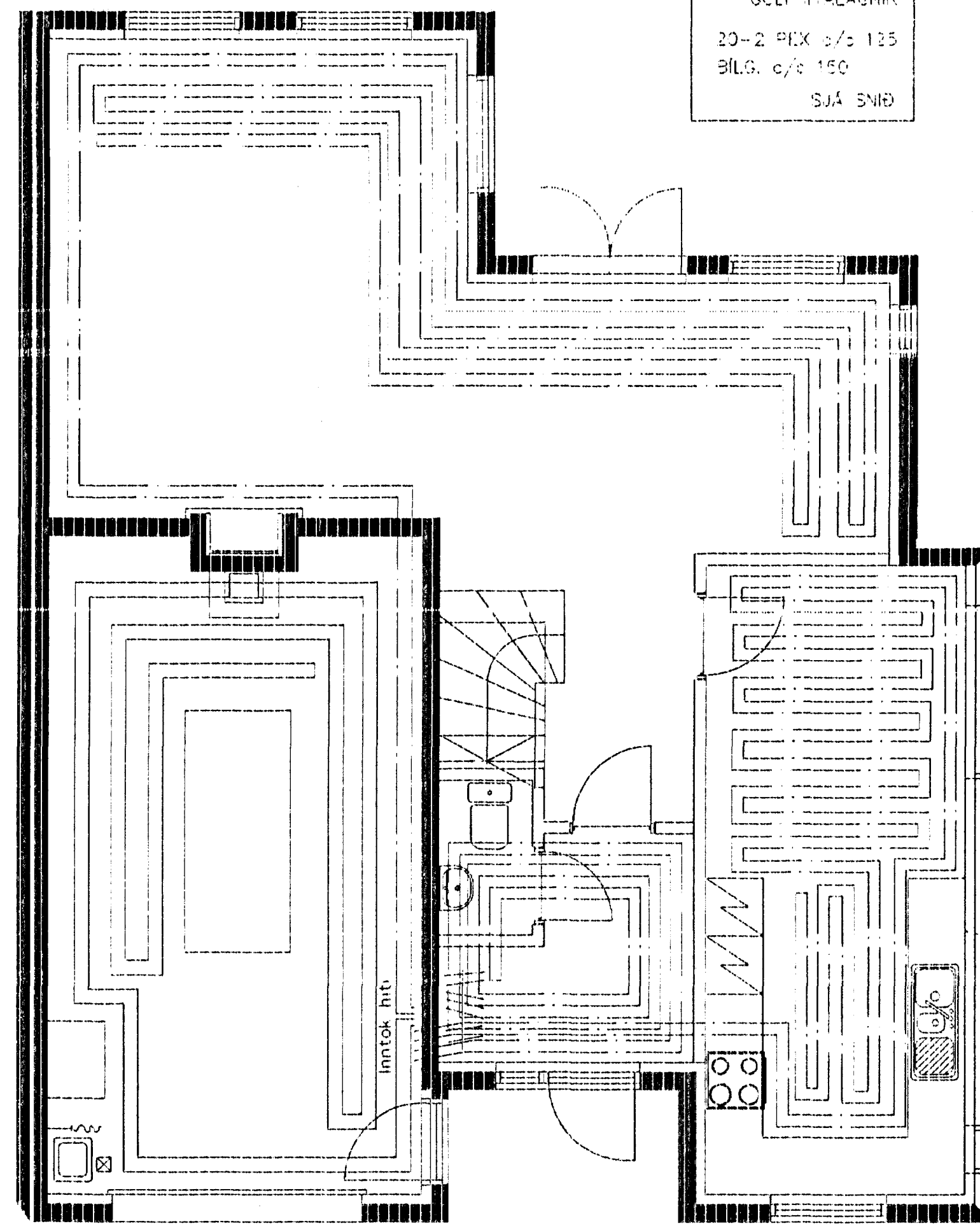
grunnmynd gölfhita
