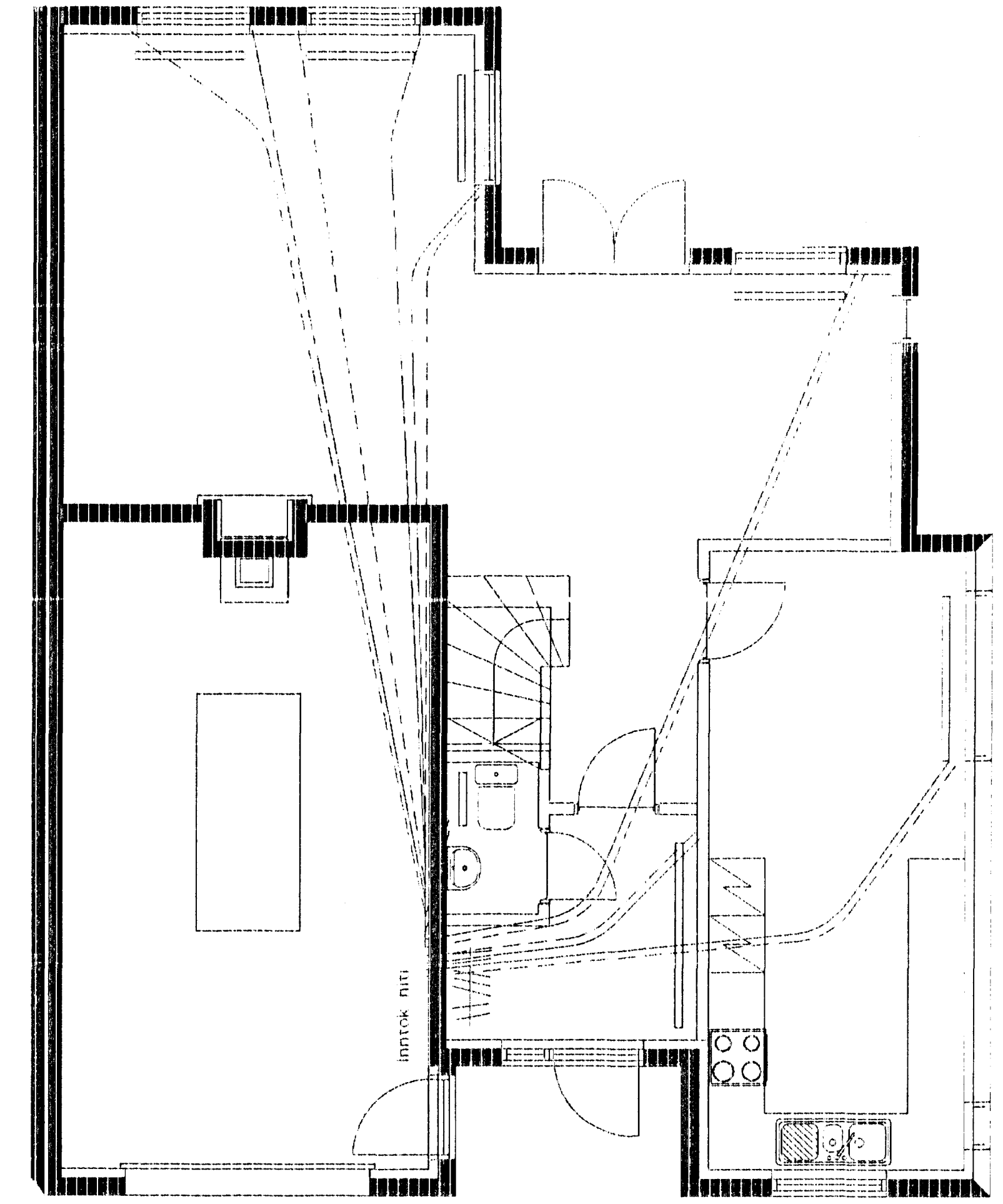
grunnmynd rör í rör ofnalagnir
