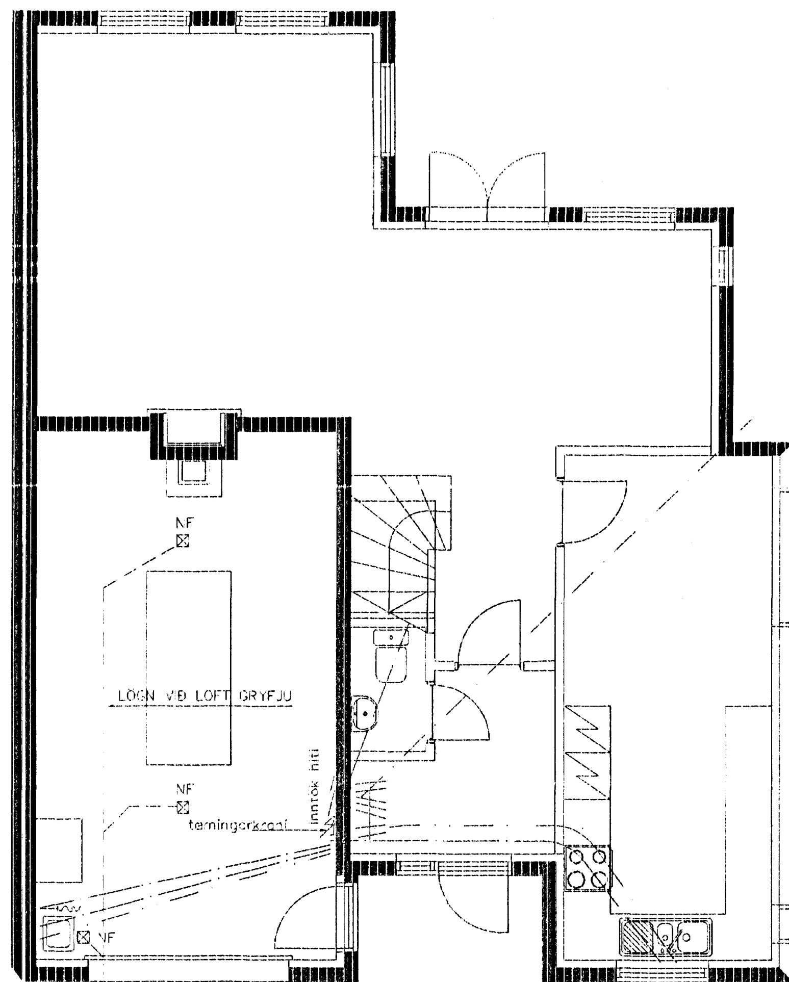
grunnmynd rör í rör neysluvatn
