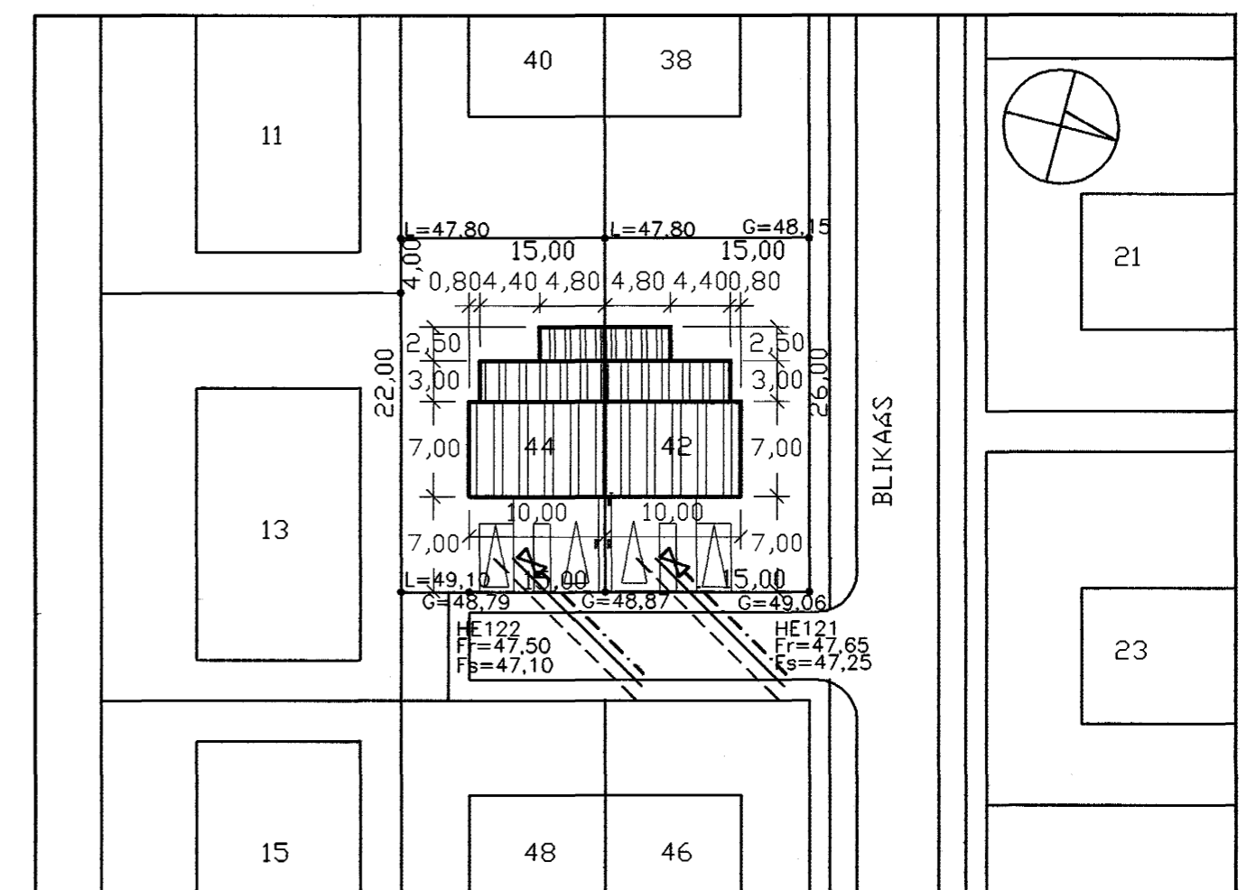
AFSTÖÐUMYND 1/500
