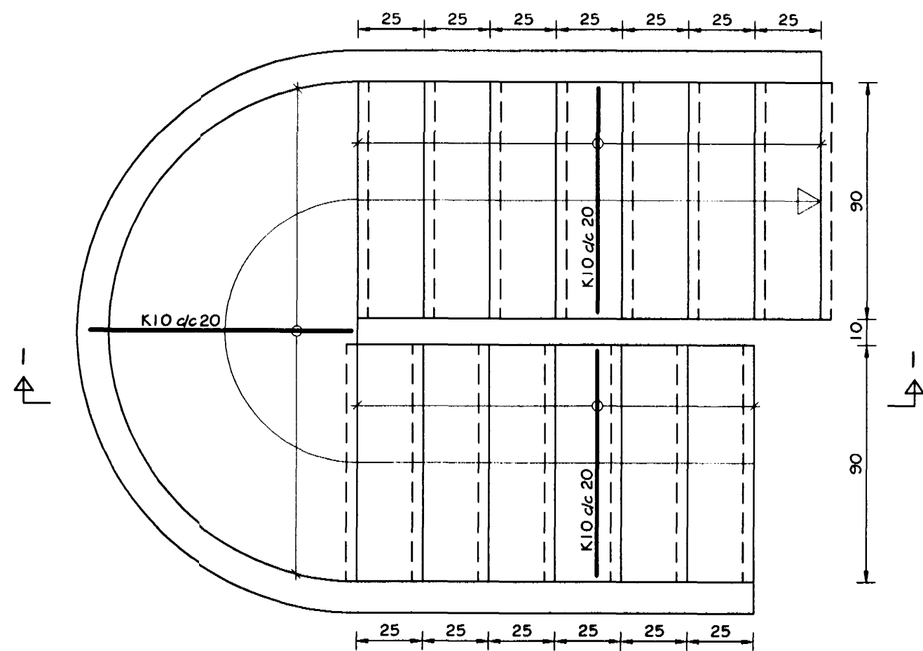
GRUNNMYND STIGA MKV. 1:20
