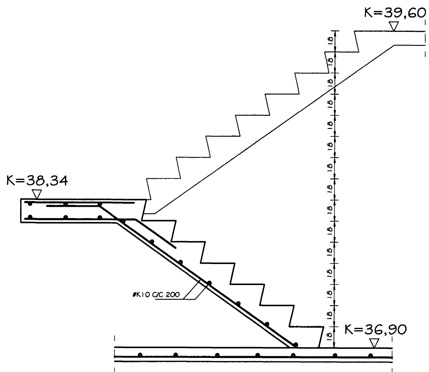
SNID I-I Í STIGA MKV. 1:20
