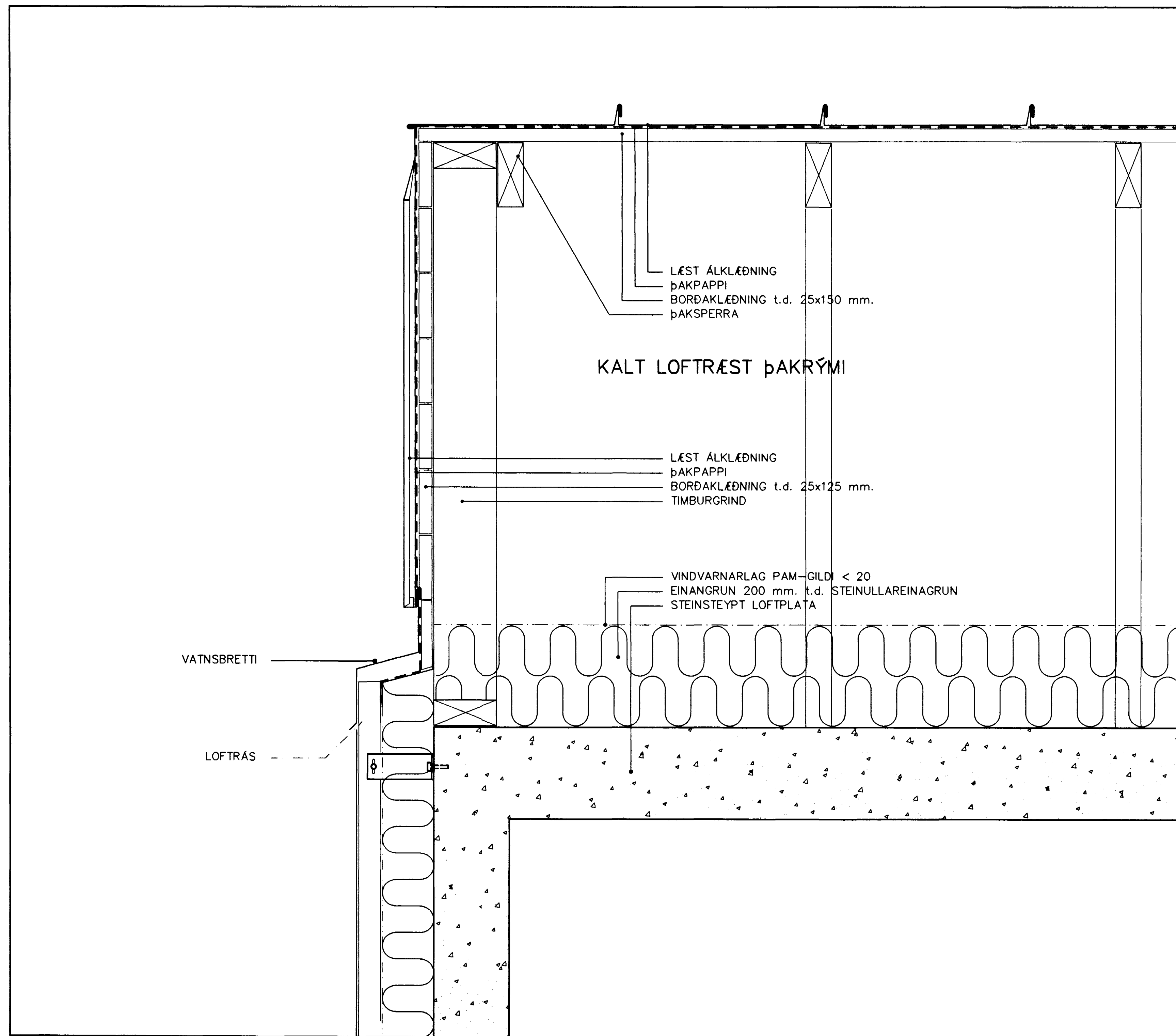
Deili 3 M.1:5
