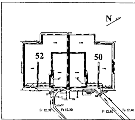
Afstöðumynd M 1:500
