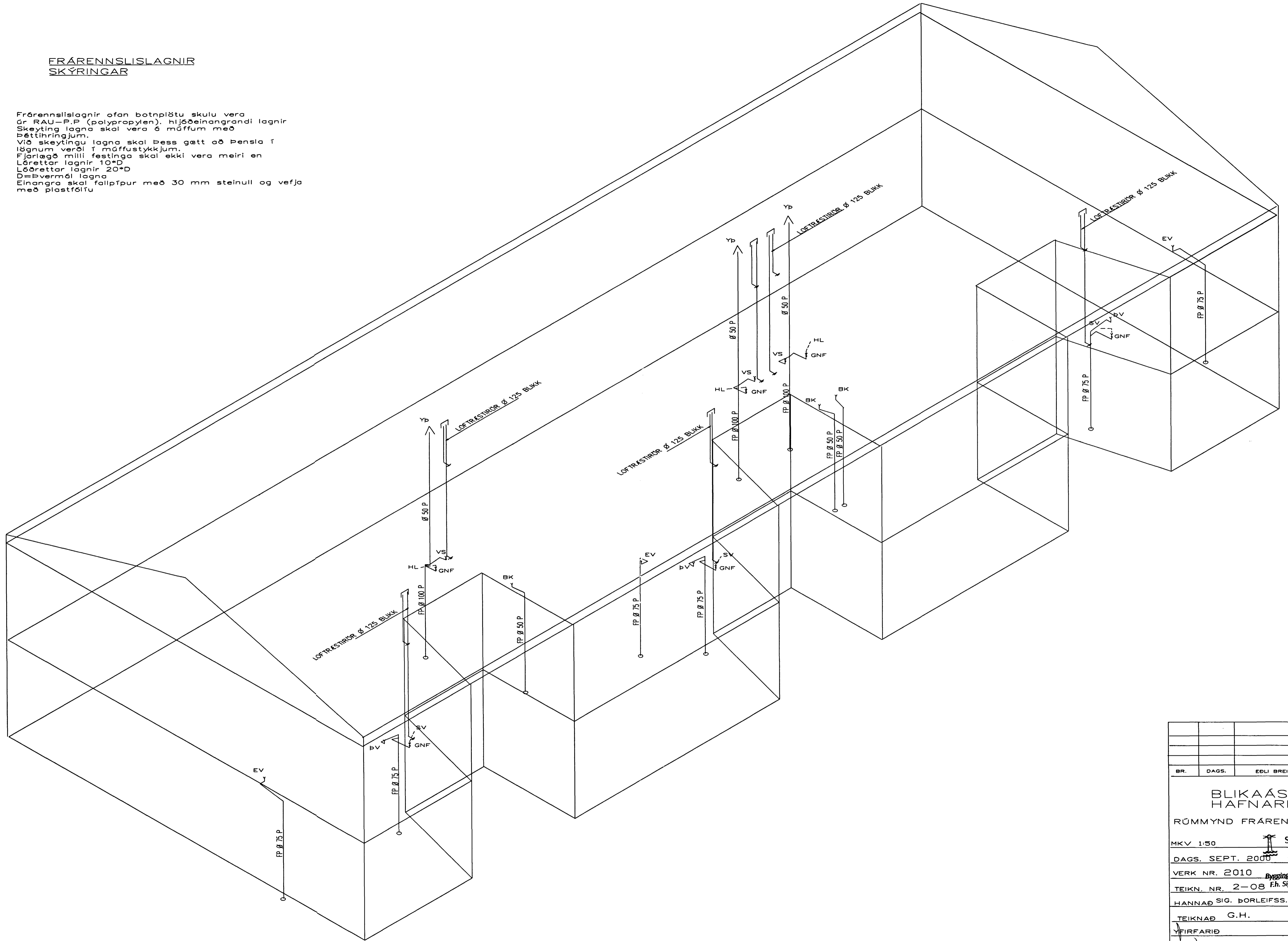
RÚMMYND FRÆRENNSLISLAGNA 1:50
