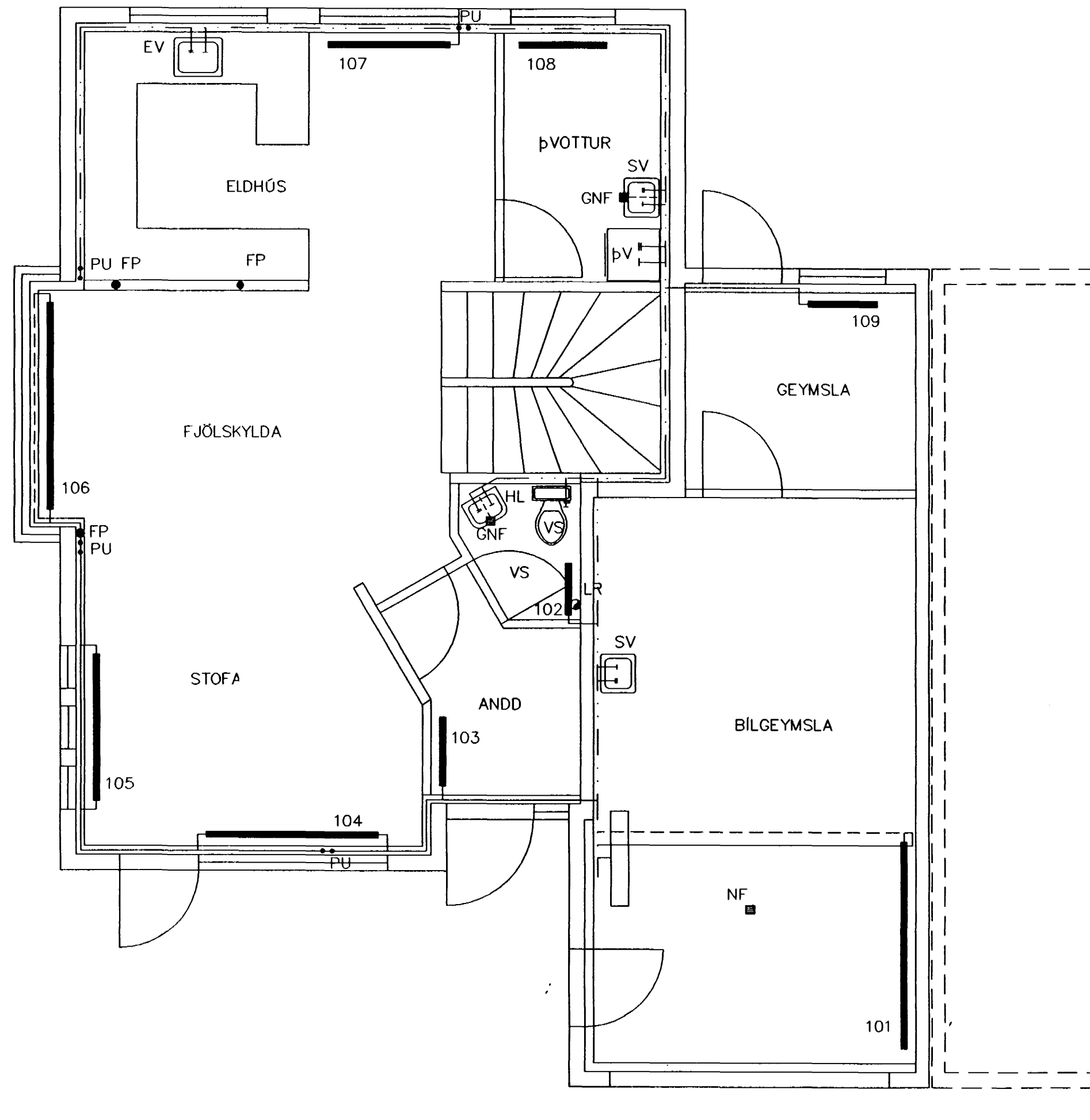
GRUNNMYND 1 HÆÐAR 1:50
