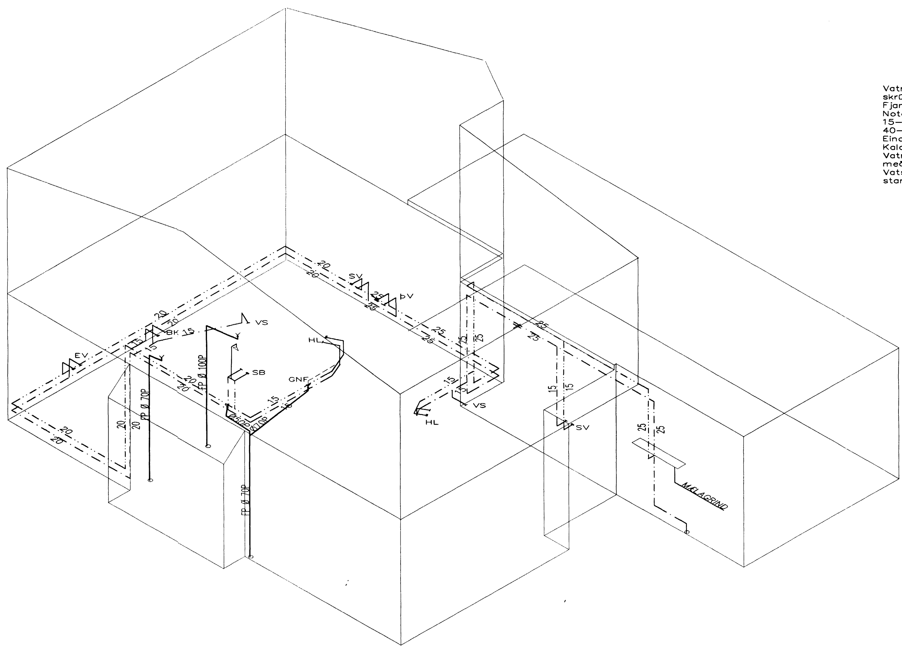
RÚMMYND VATNS OG FRÁRENNSLISLAGNA 1:50
