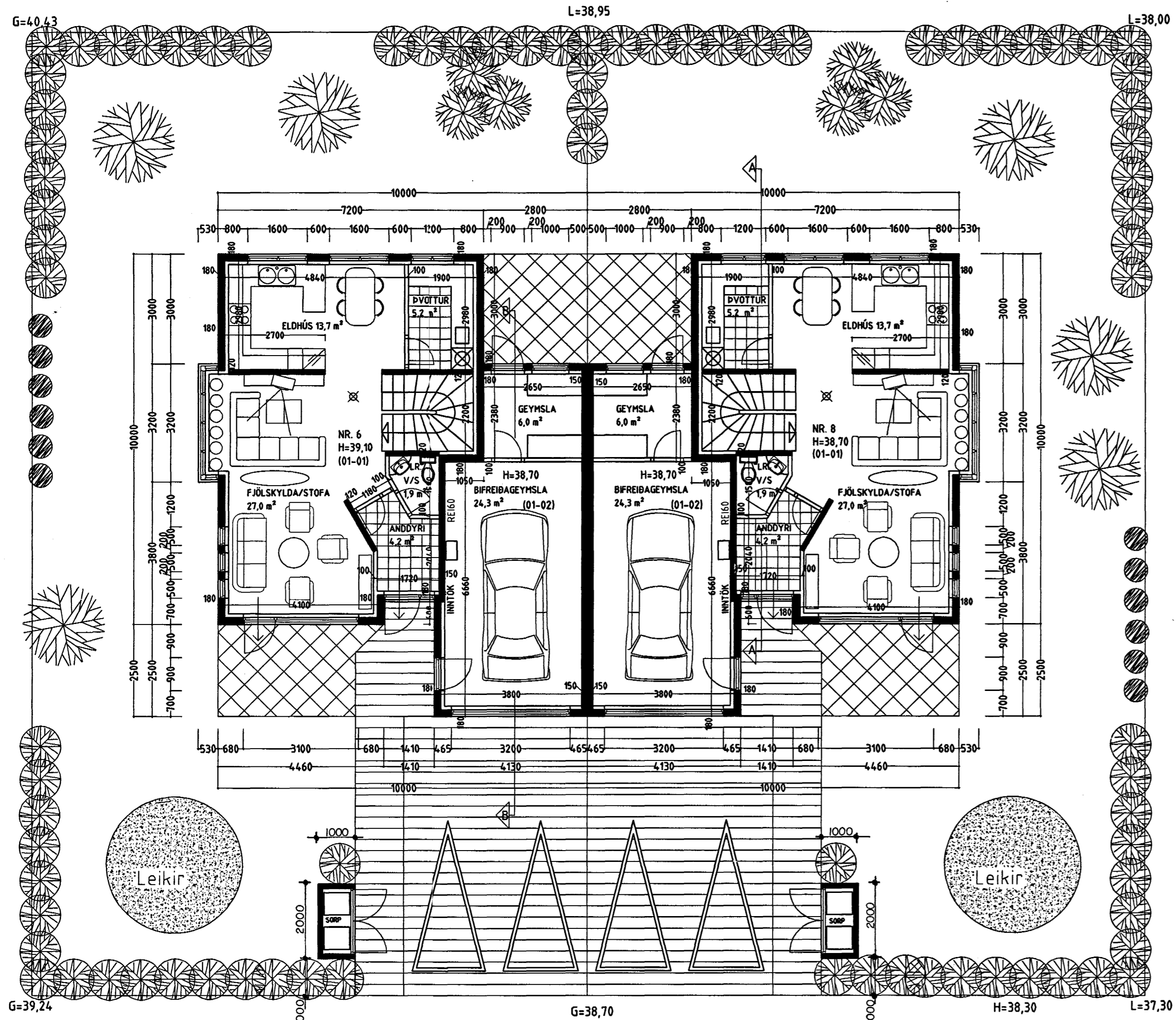
GRUNNMYND 1 HÆÐ MKV. 1:100.
