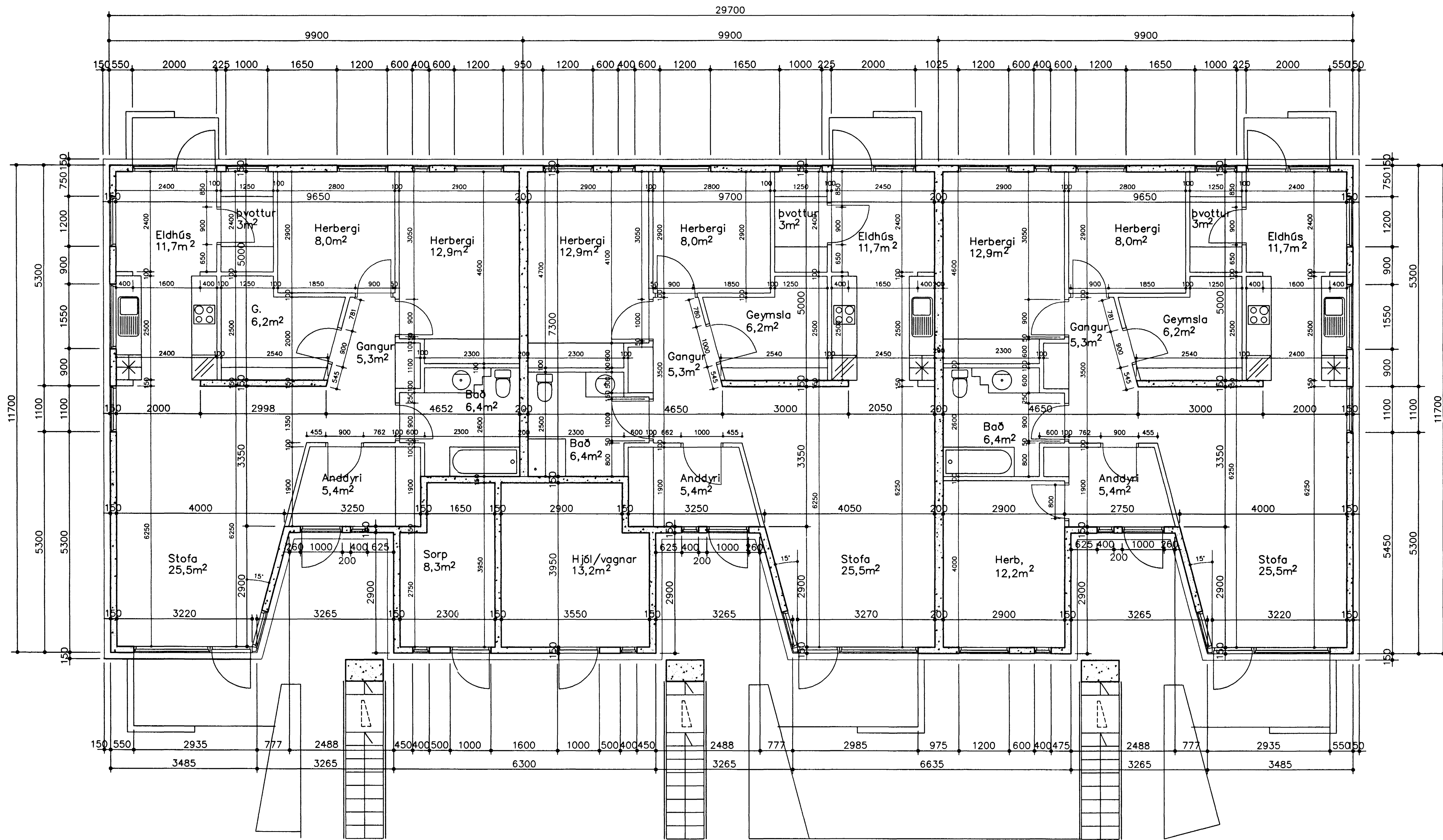
Grunnmynd 1.hæð
