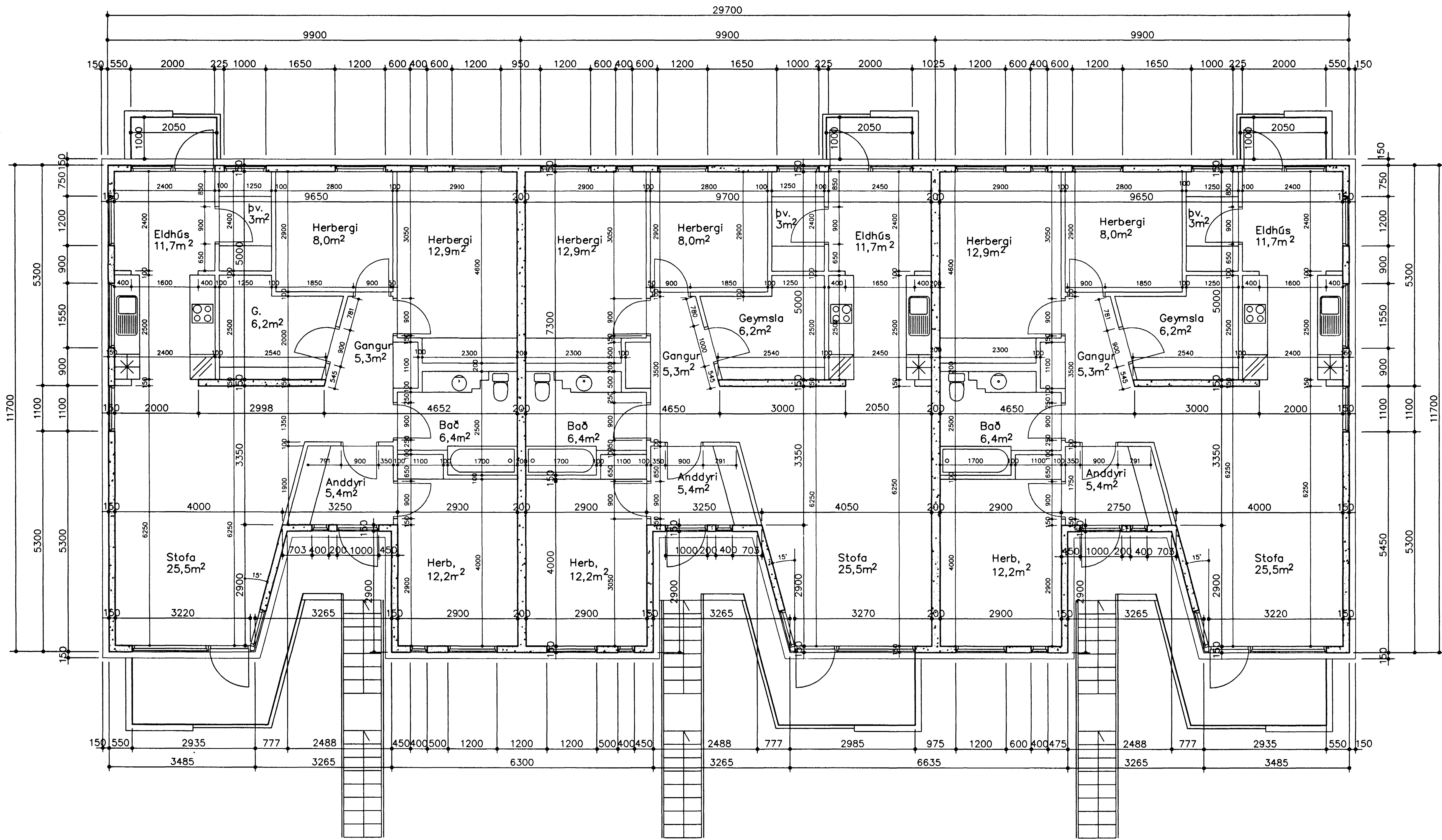
Grunnmynd 2.hæð
