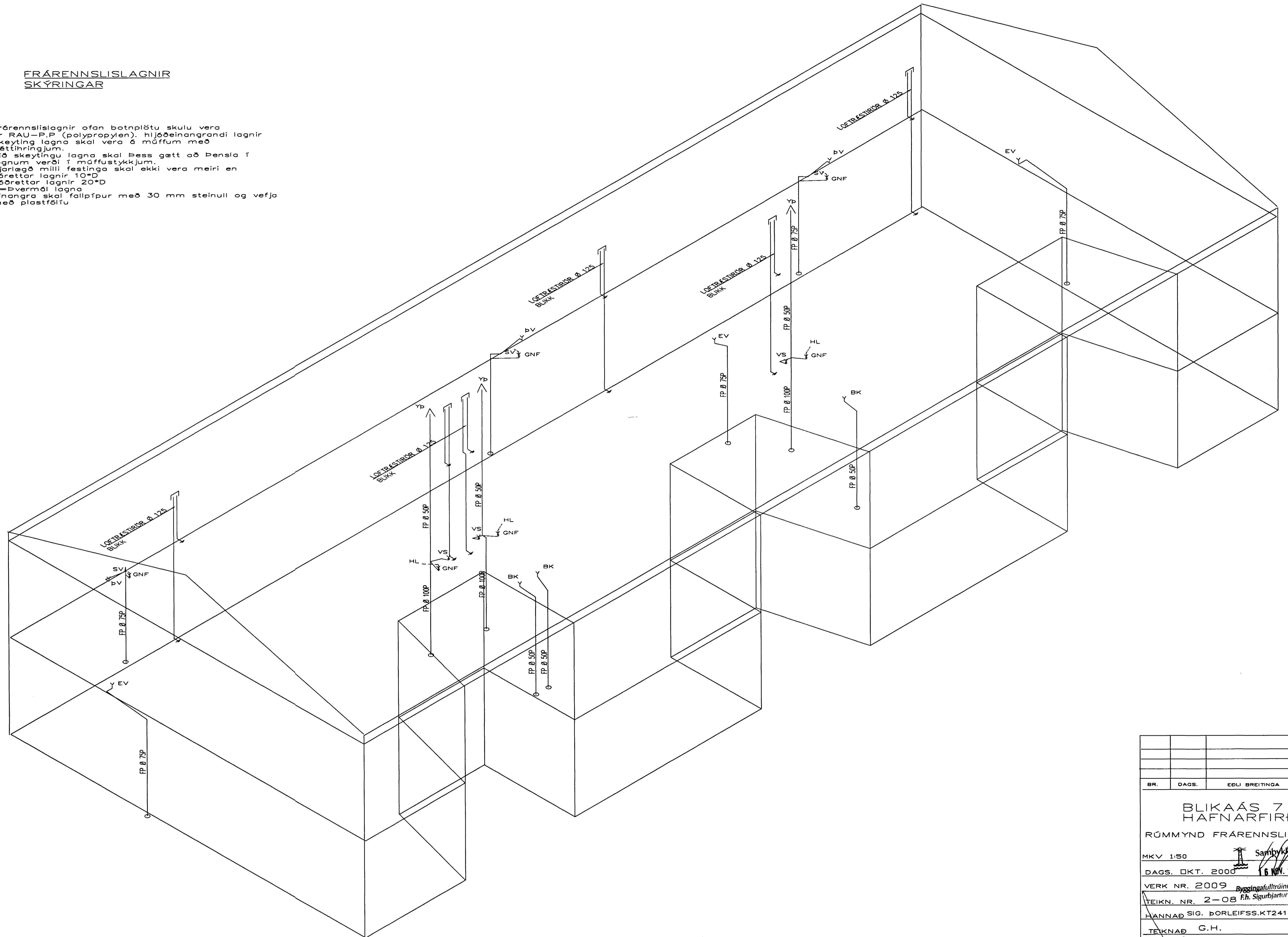
RÚMMYND FRÆRENNSLISLAGNA 1:50
