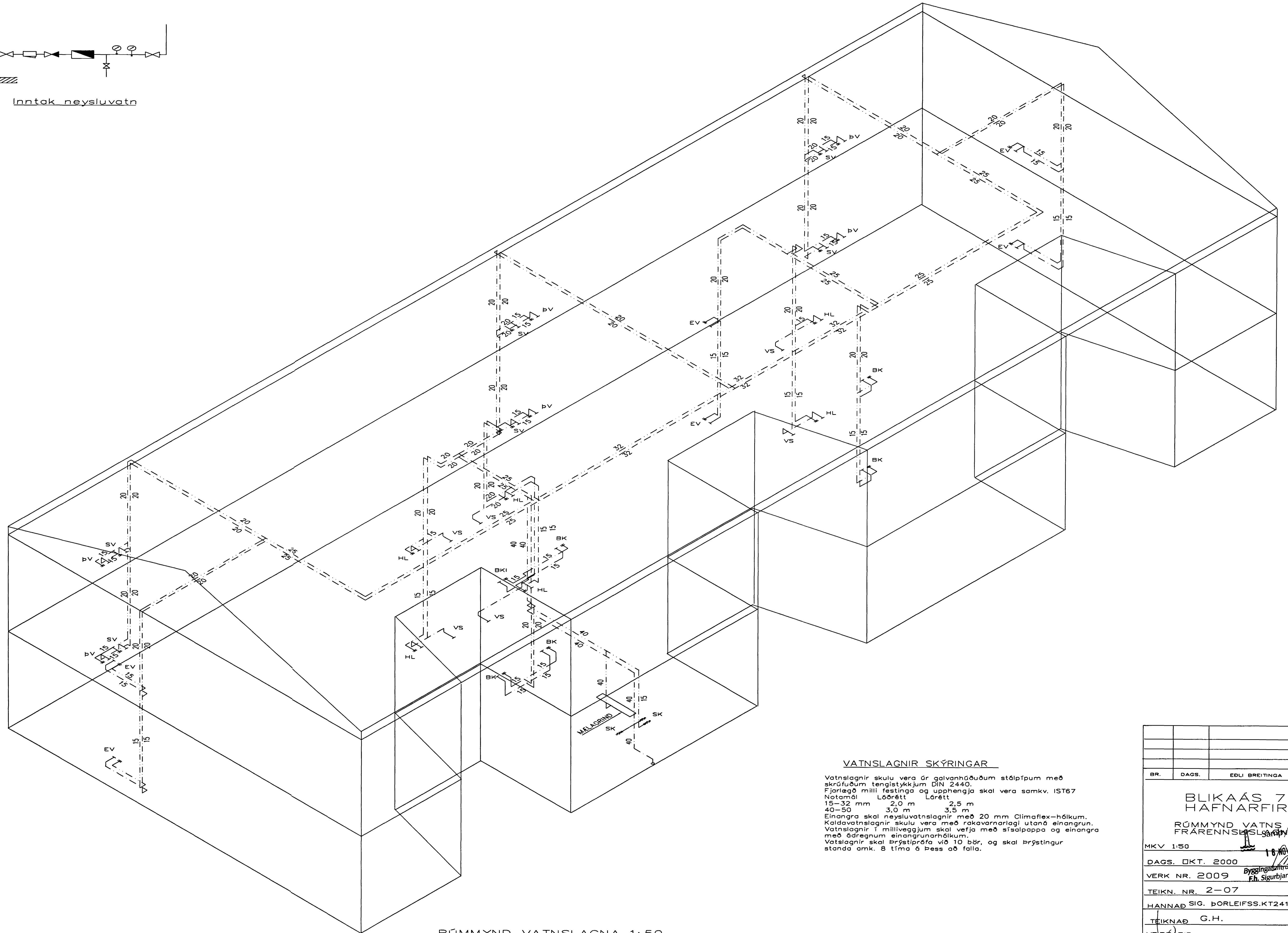
RÚMMYND VATNSLAGNA 1:50
