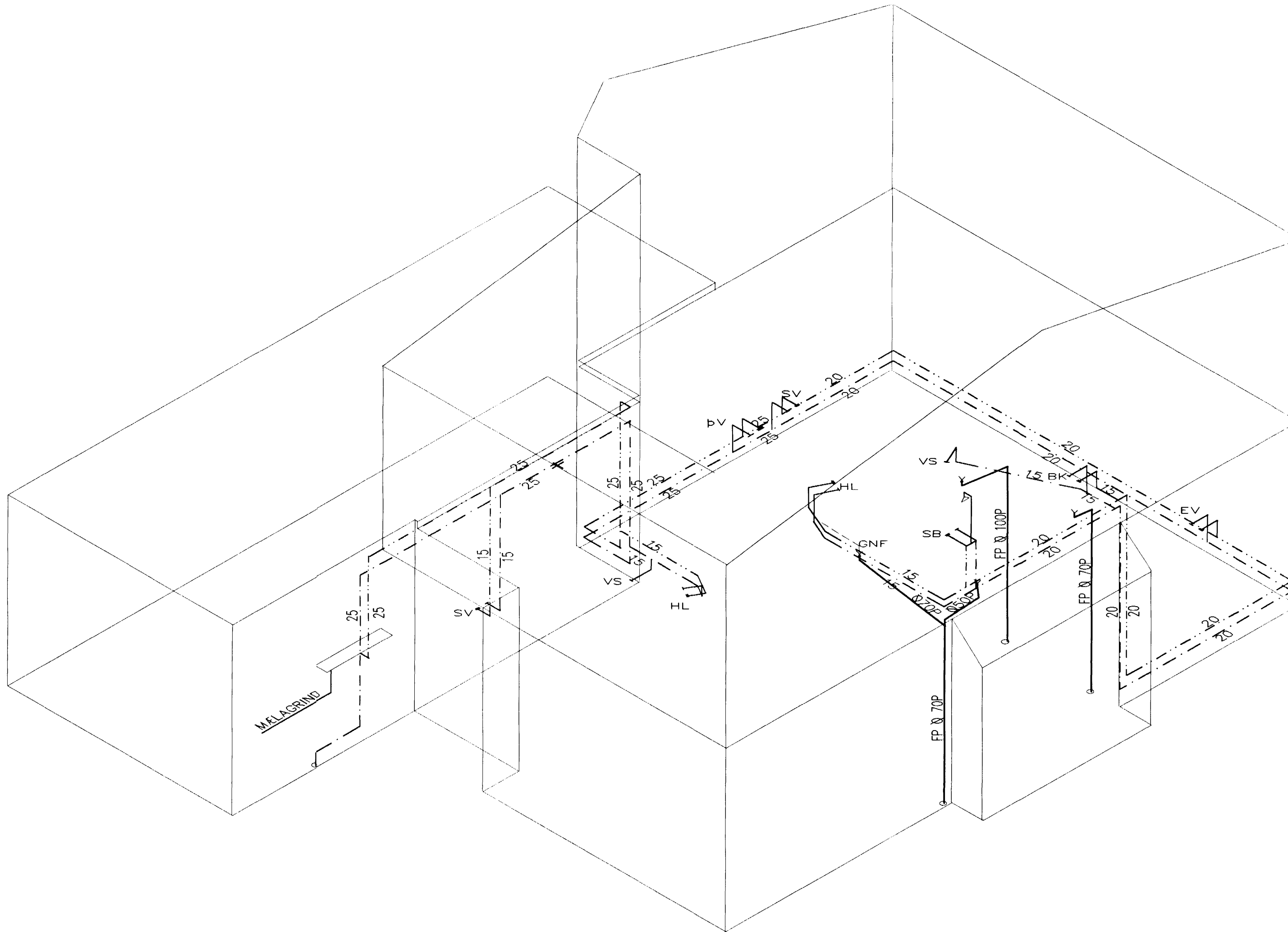
RÚMMYND VATNS OG FRÁRENNSLISLAGNA 1:50
