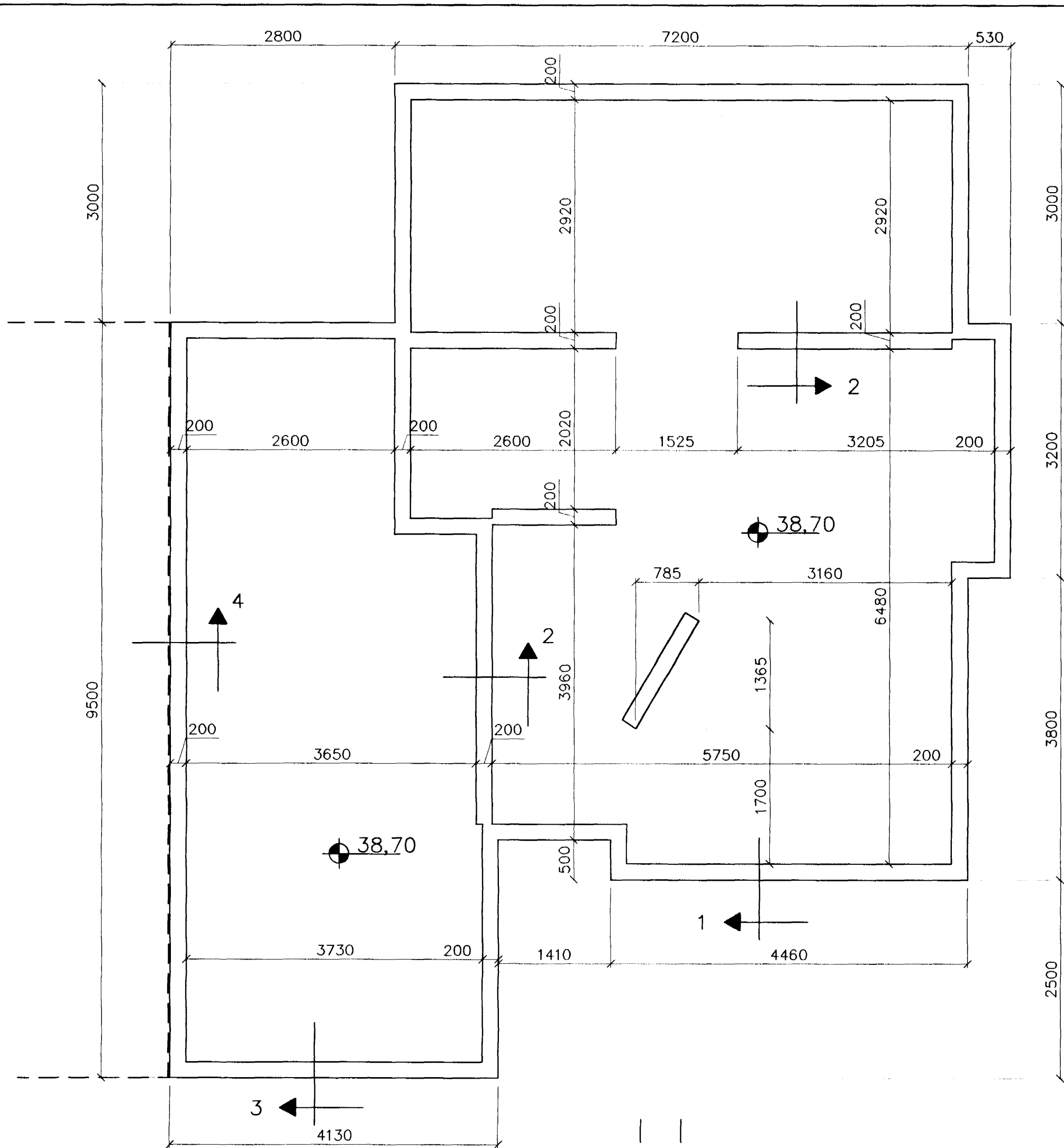
Grunnmynd, 1:50
