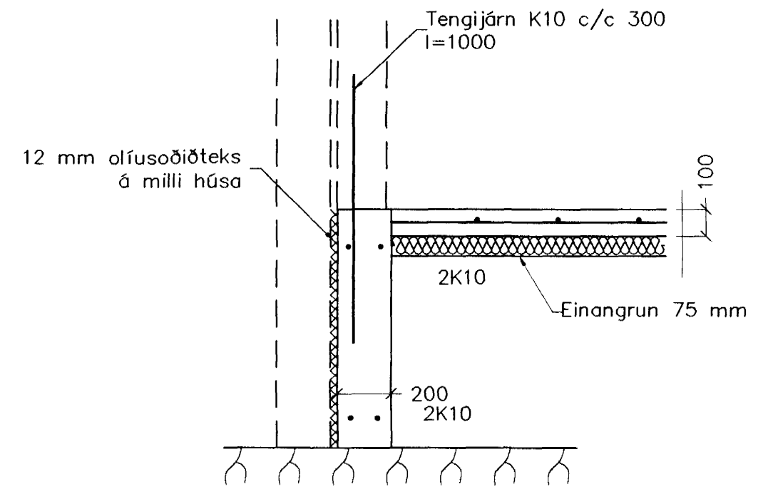
Snið 4, 1:20
