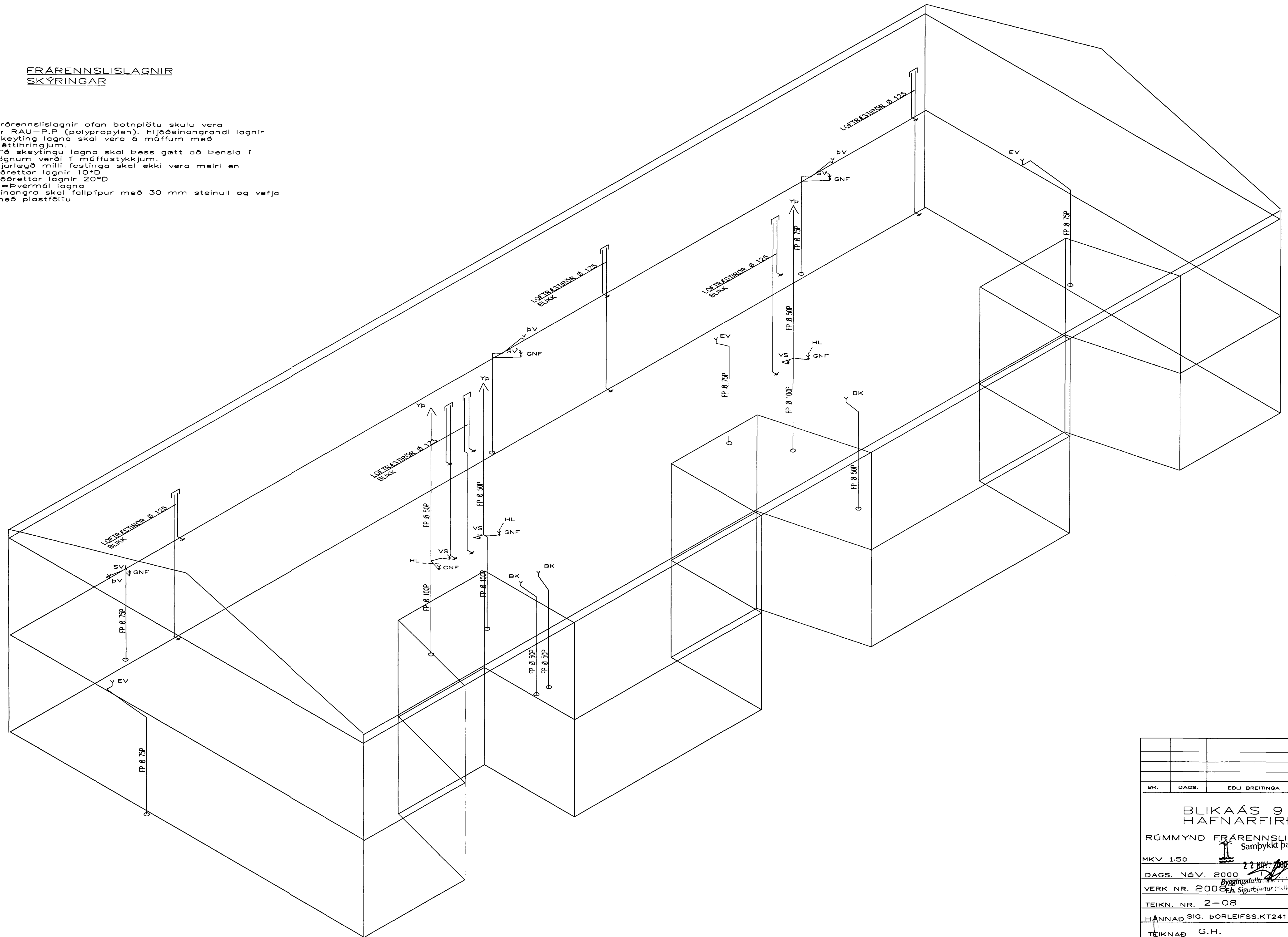
RÚMMYND FRÆRENNSLISLAGNA 1:50
