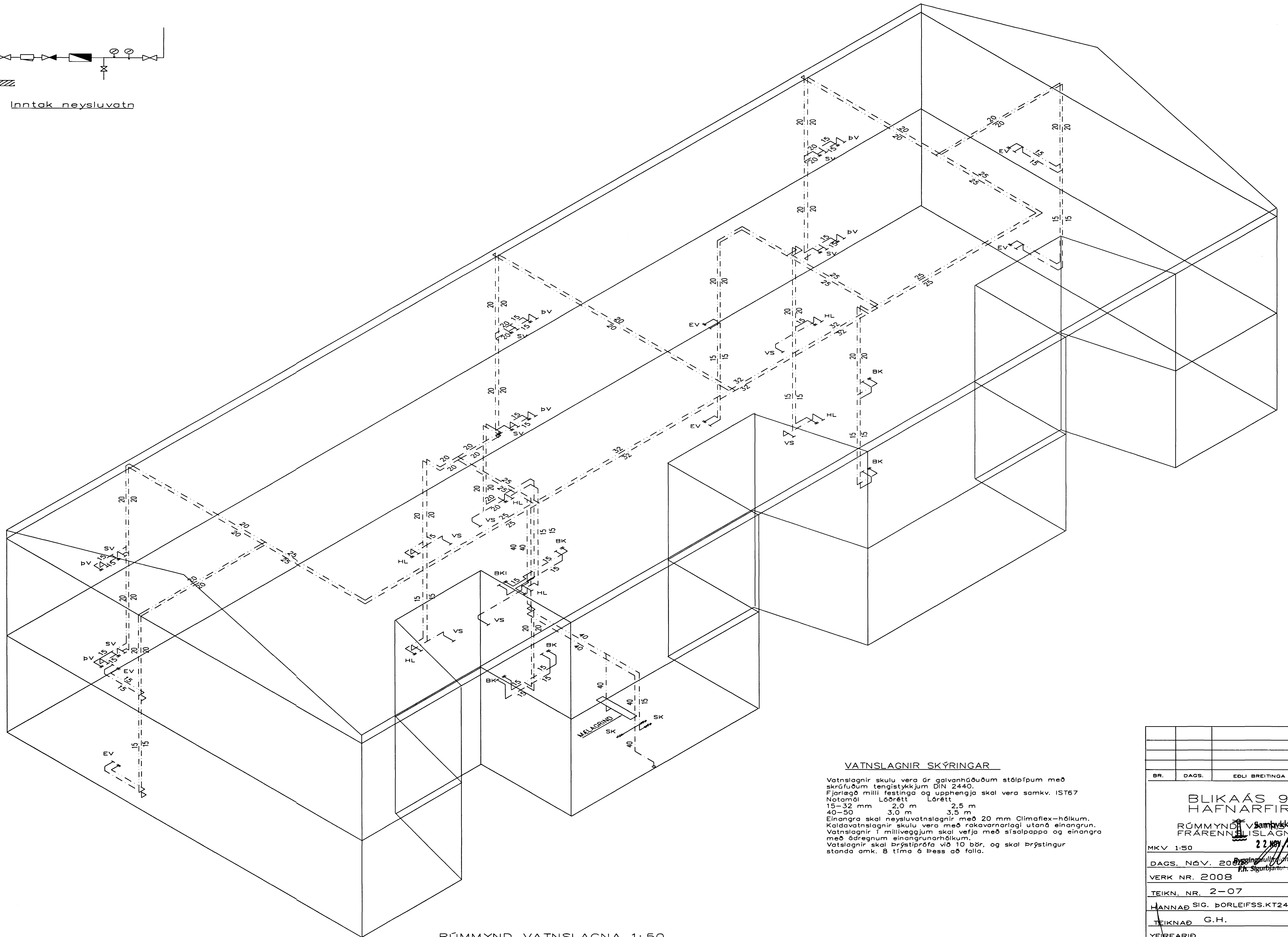
RÜMMYND VATNSLAGNA 1:50
