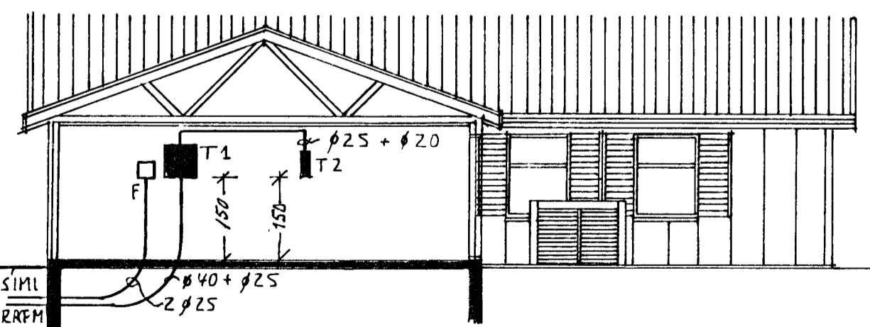
SKURÐUR M 1:100
