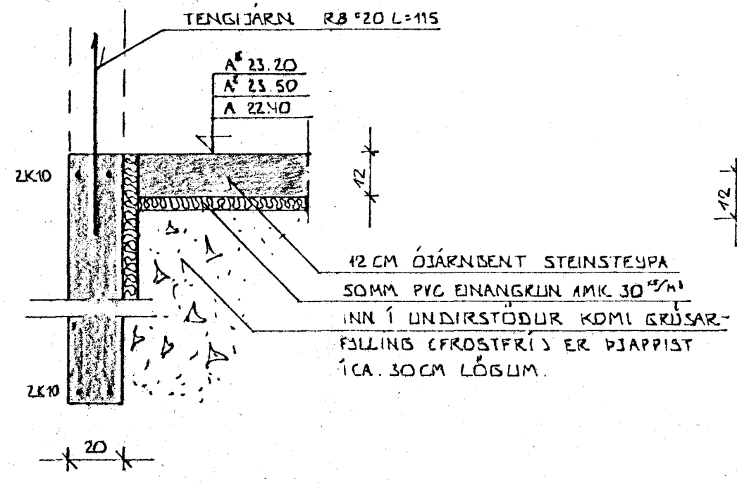
SNID A-A í ÚTVEGG 1:20
