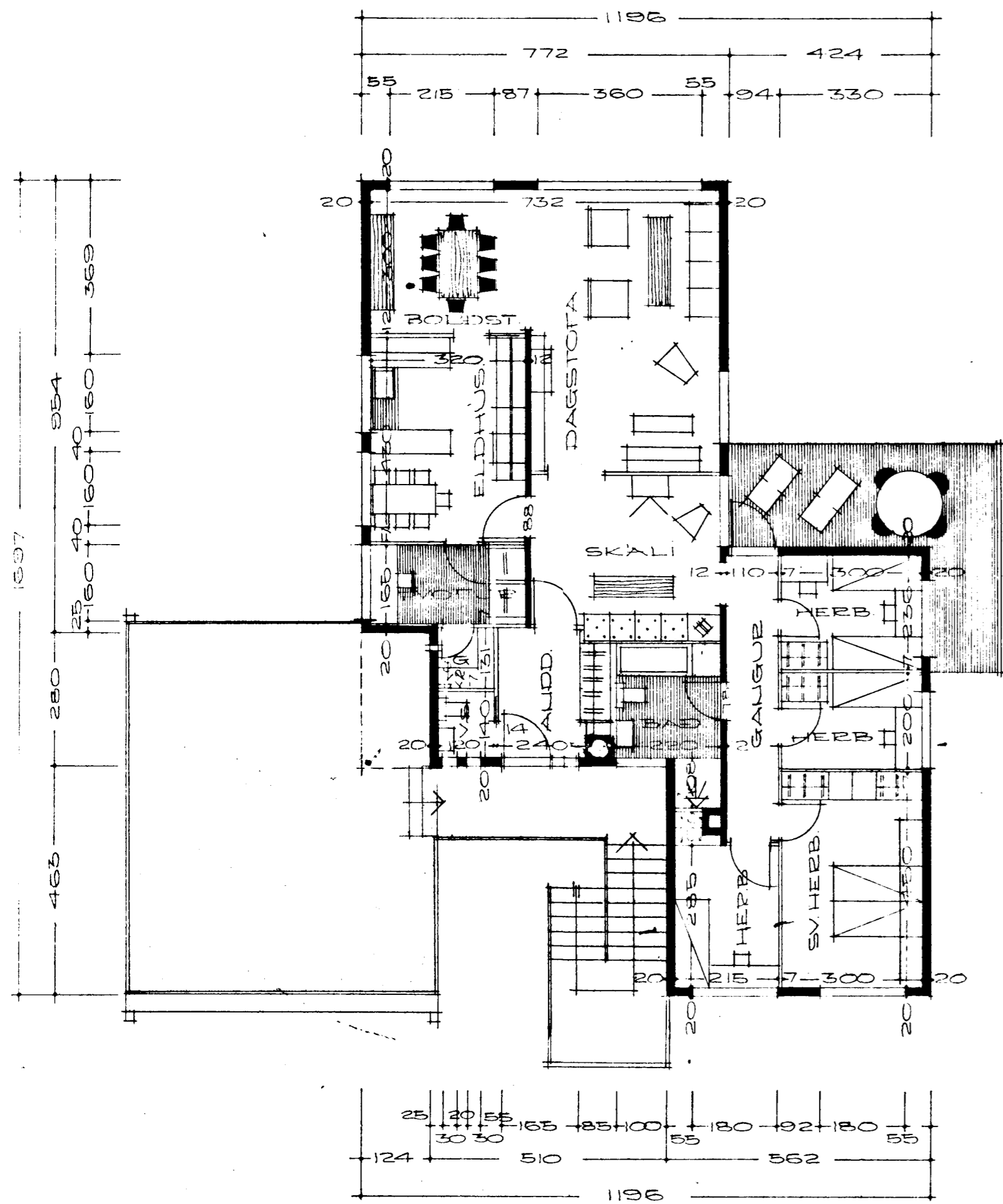
2 HÆÐ.
