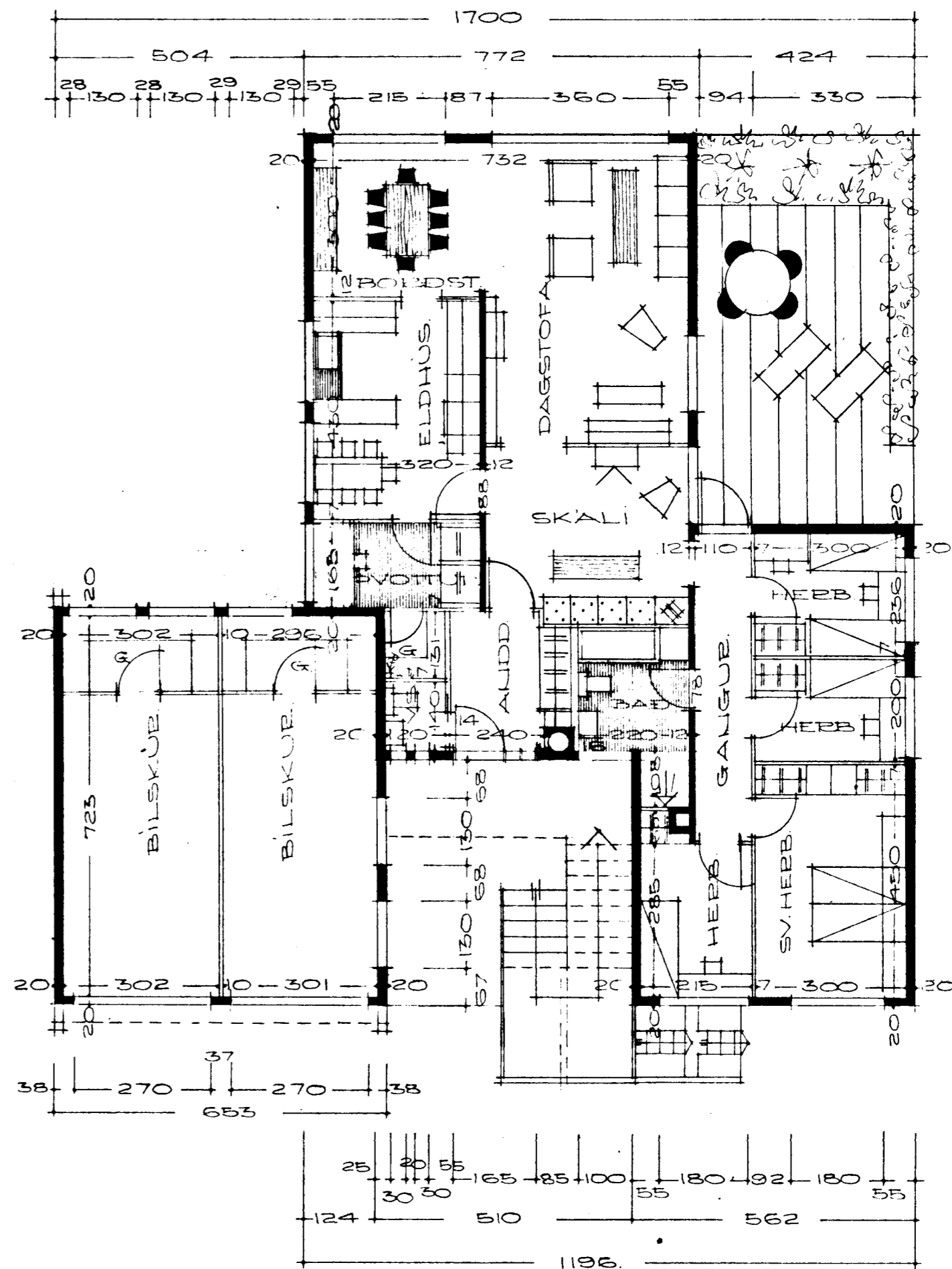
1. HÆÐ
