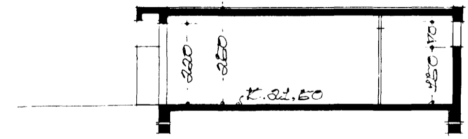
STURÐUR B-B
