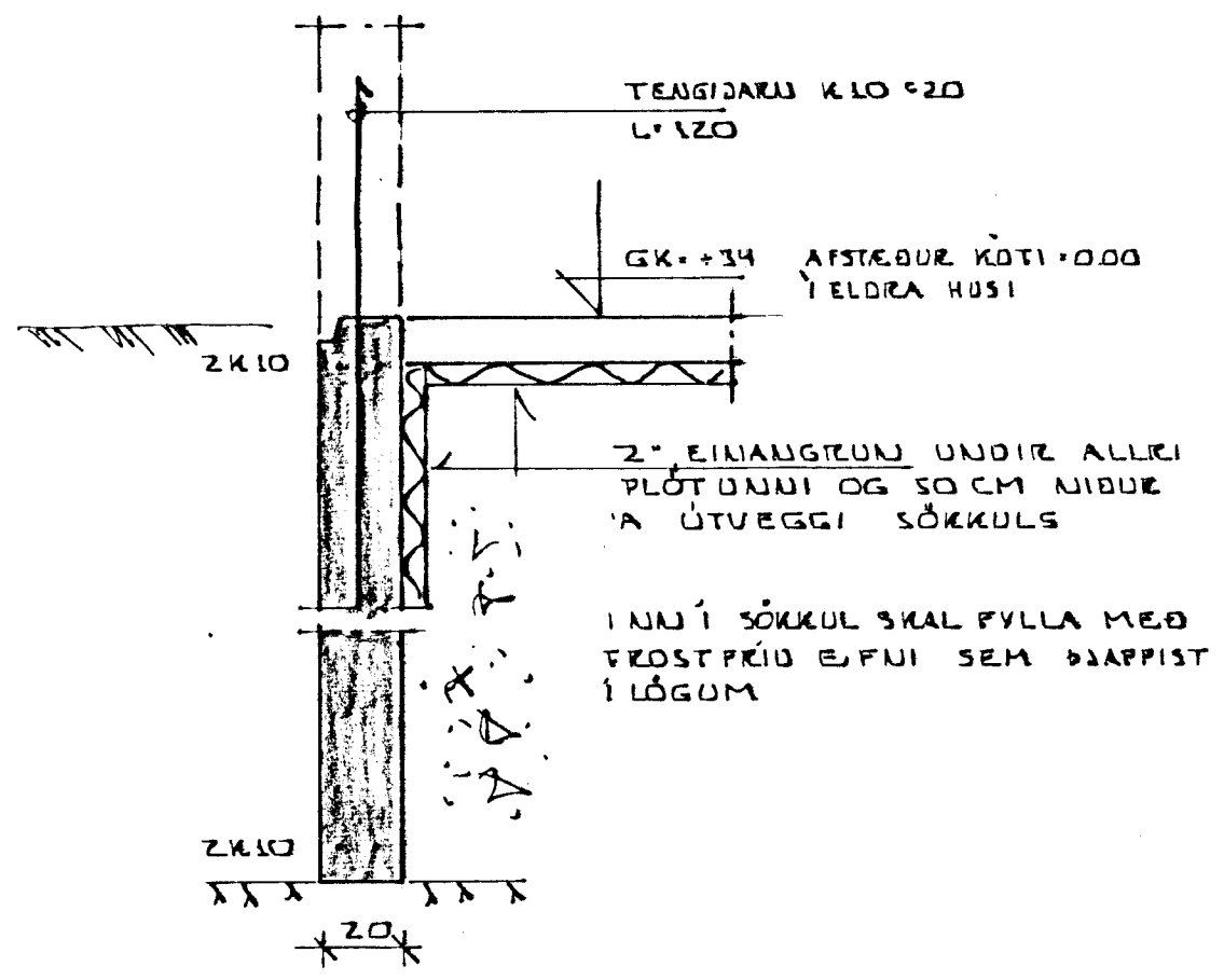
SNID I UNDIRSTÖÐUR 1:20
