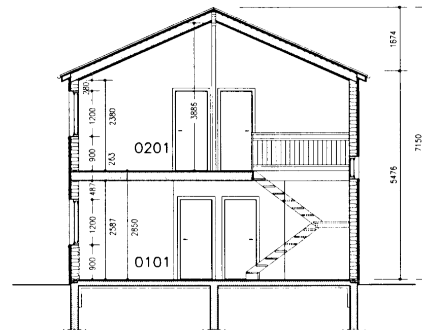
SNID 1-1 1:100
