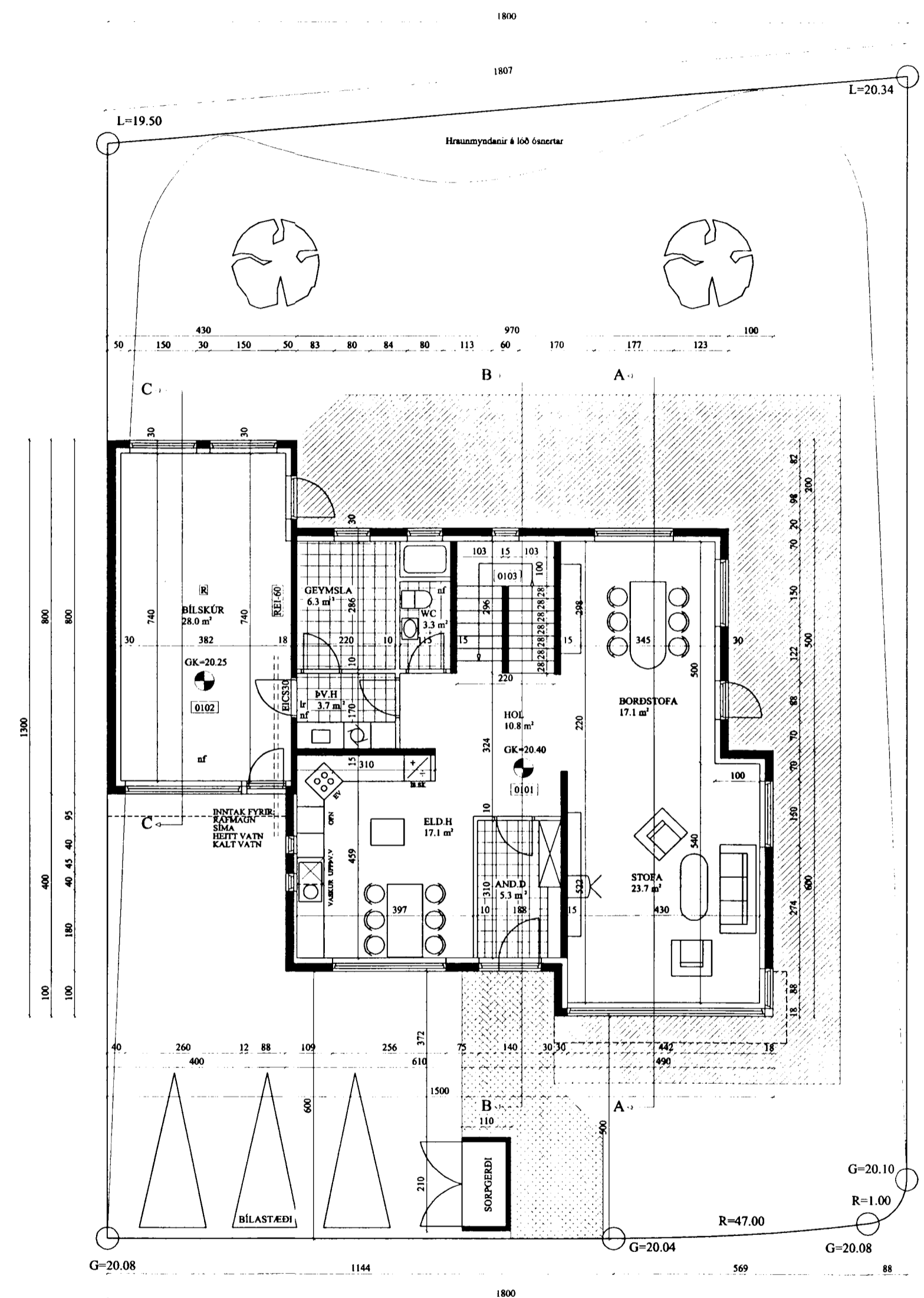
GRUNNMYND 1.HÆÐ.
