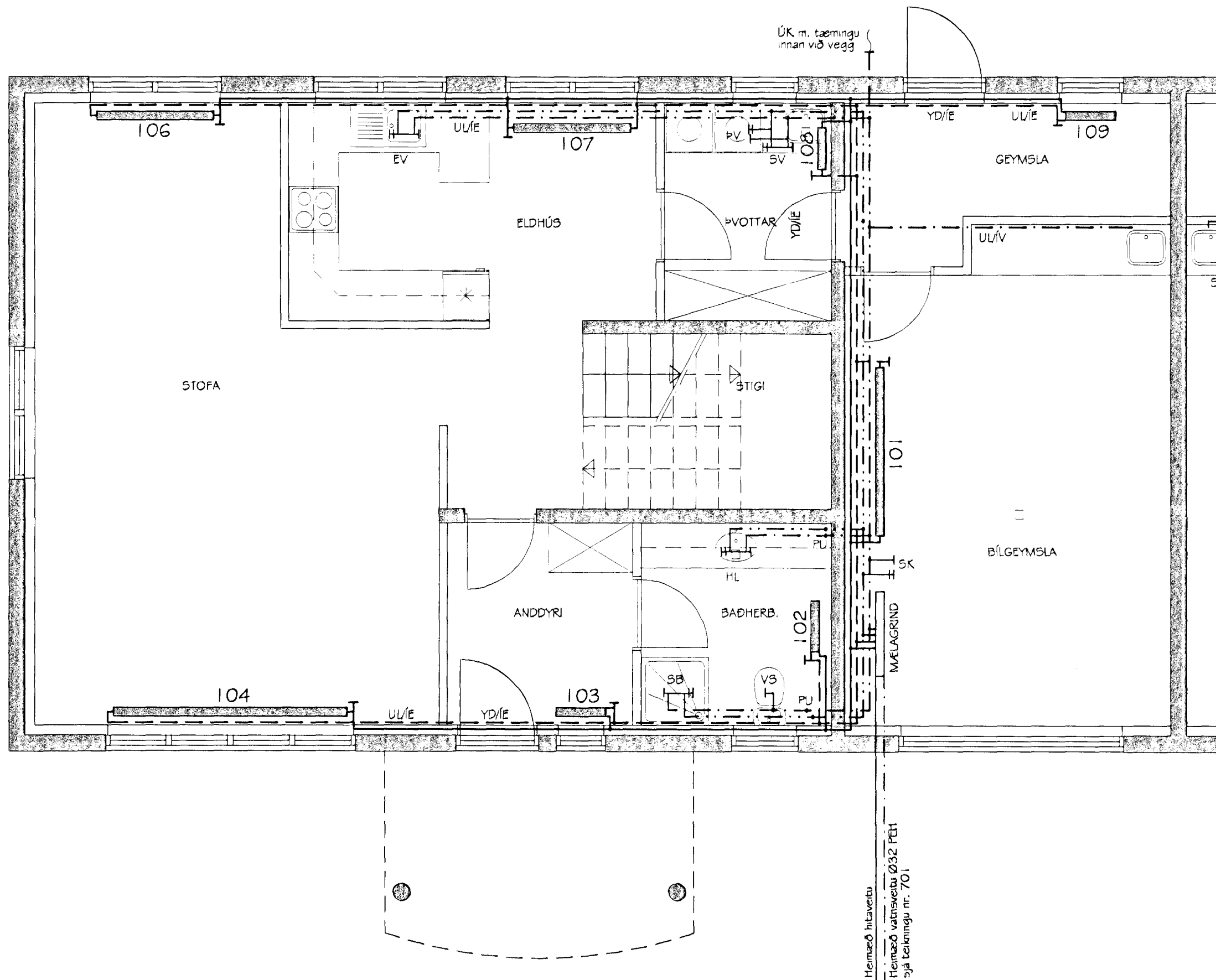
BLÓMVELLIR 27 HITA- OG NEYSLUVATNSLAGNIR GRUNNMYND NEDRI HÆÐAR MKV. 1:50
