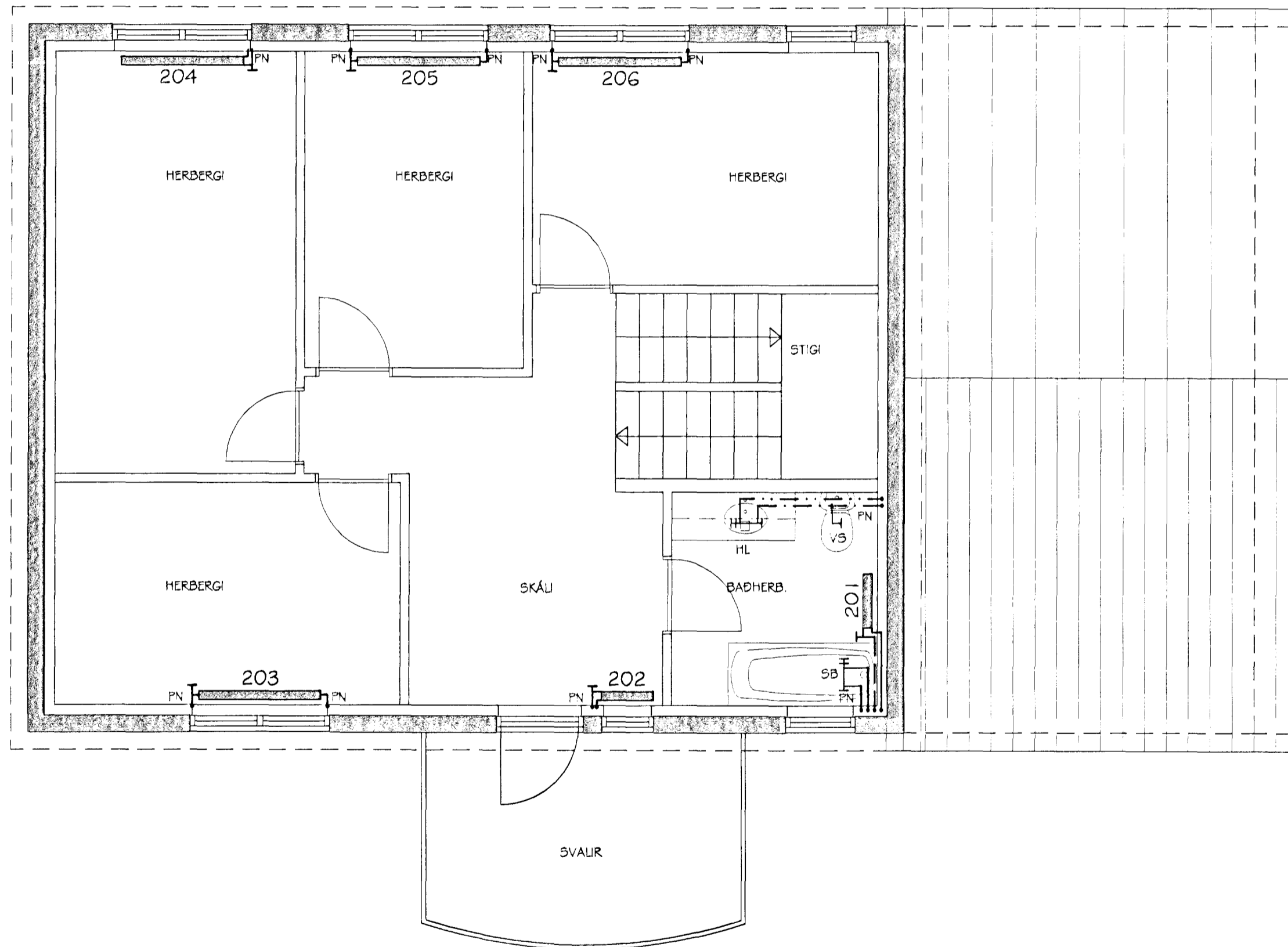
BLÓMVELLIR 27 HITÁ- OG NEYSLUVATNSLAGNIR GRUNNMYND NEÐRI HÆÐAR MKV. 1:50
