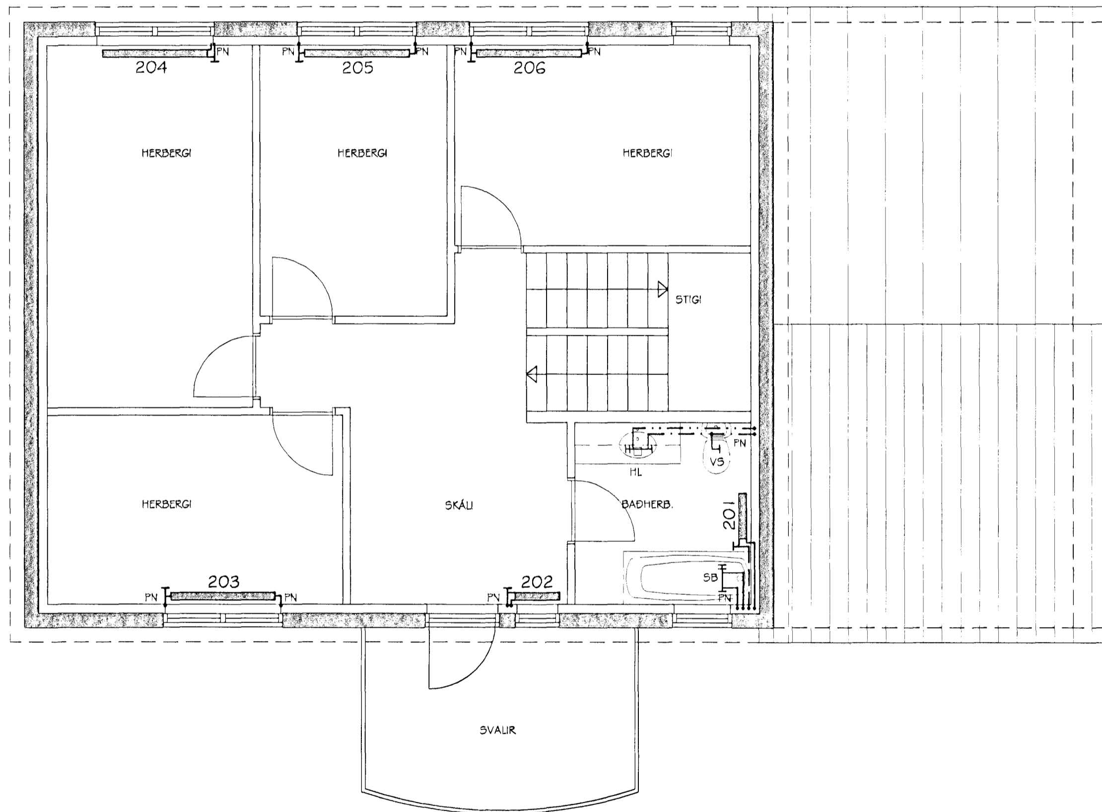
BLÓMVELLIR 27 HITA- OG NEYSLUVATNSLAGNIR GRUNNMYND NEDRI HÆÐAR MKV. 1:50
