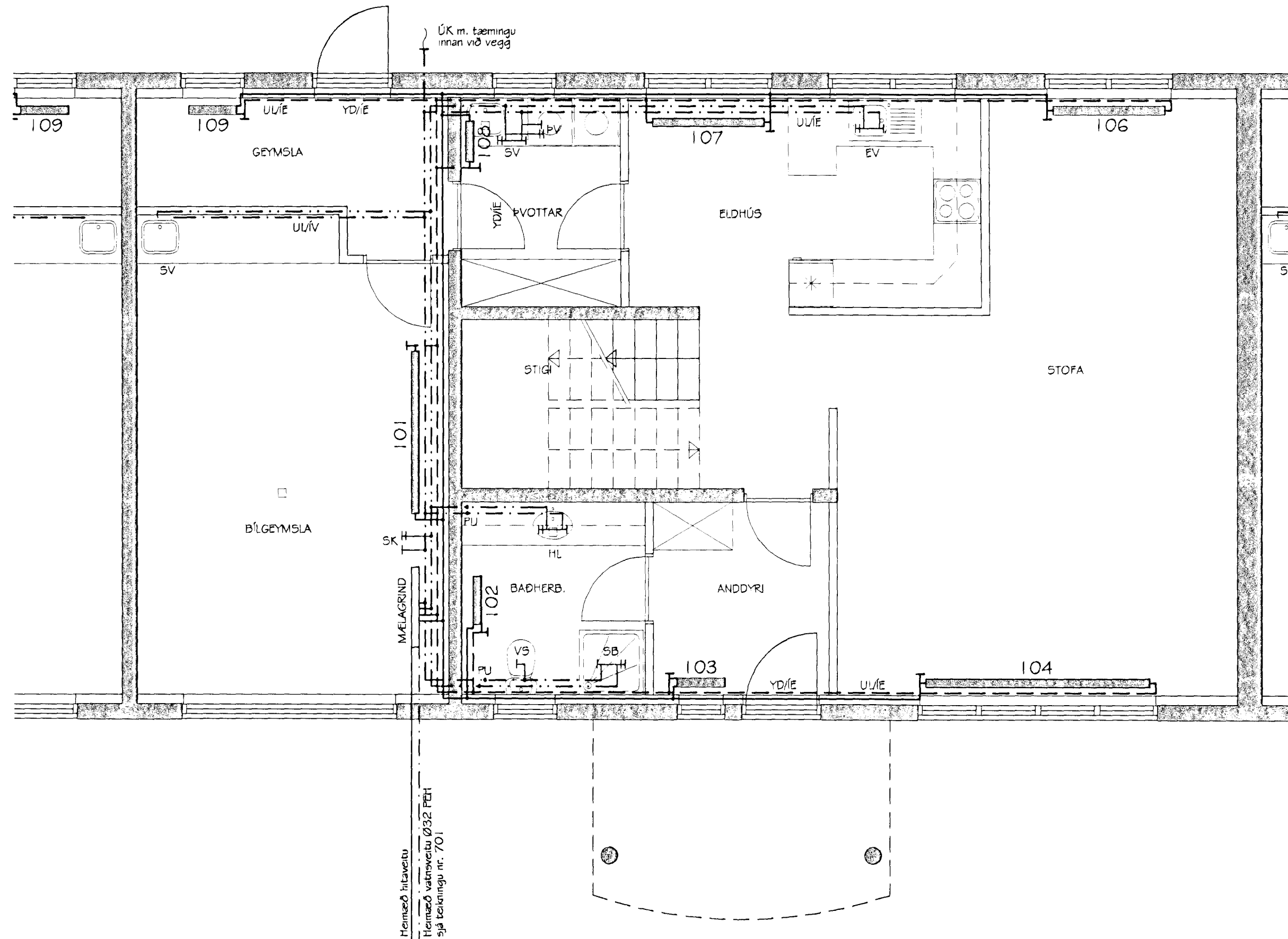
BLÓMVELLIR 29 HIT- OG NEYSLUVATNSLAGNIR GRUNNMYND NEDRI HÆÐAR MKV. 1:50
