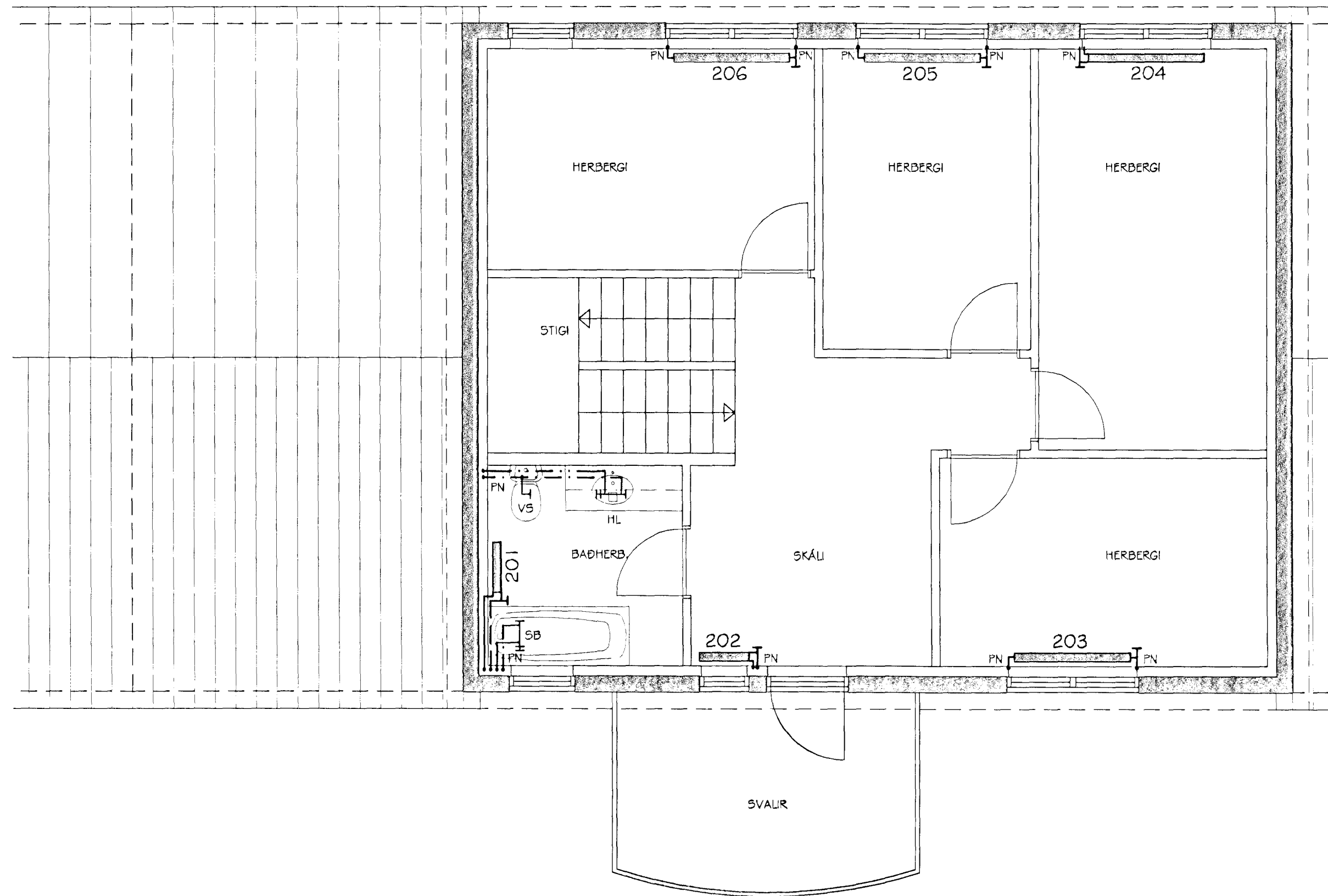
BLÓMVELLIR 29 HITA- OG NEYSLUVATNSLAGNIR GRUNNMYND NEDRI HÆÐAR MKV. 1:50
