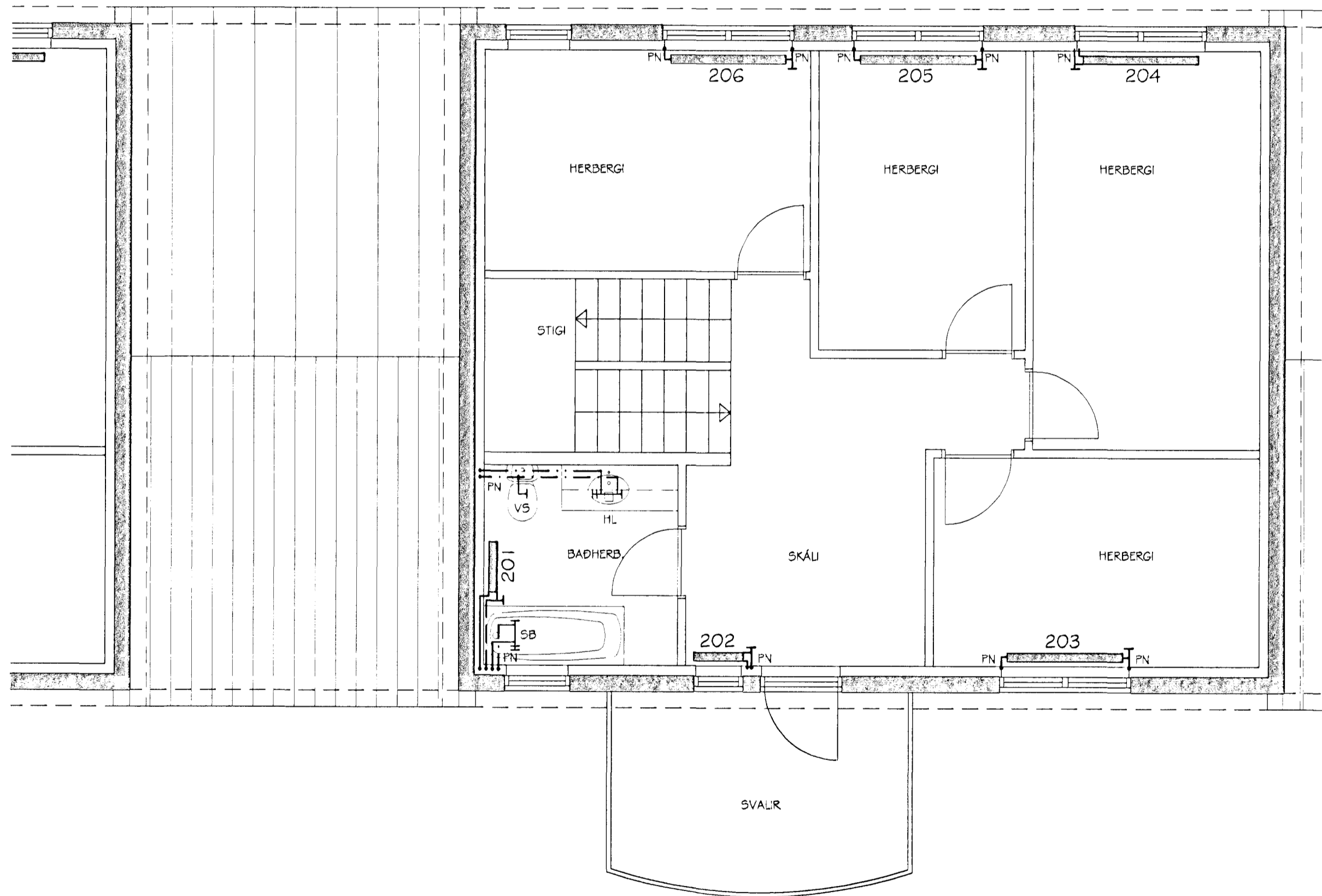
BLÓMVELLIR 31 HITA- OG NEYSLUVATNSLAGNIR GRUNNMYND NEDRI HÆÐAR MKV. 1:50
