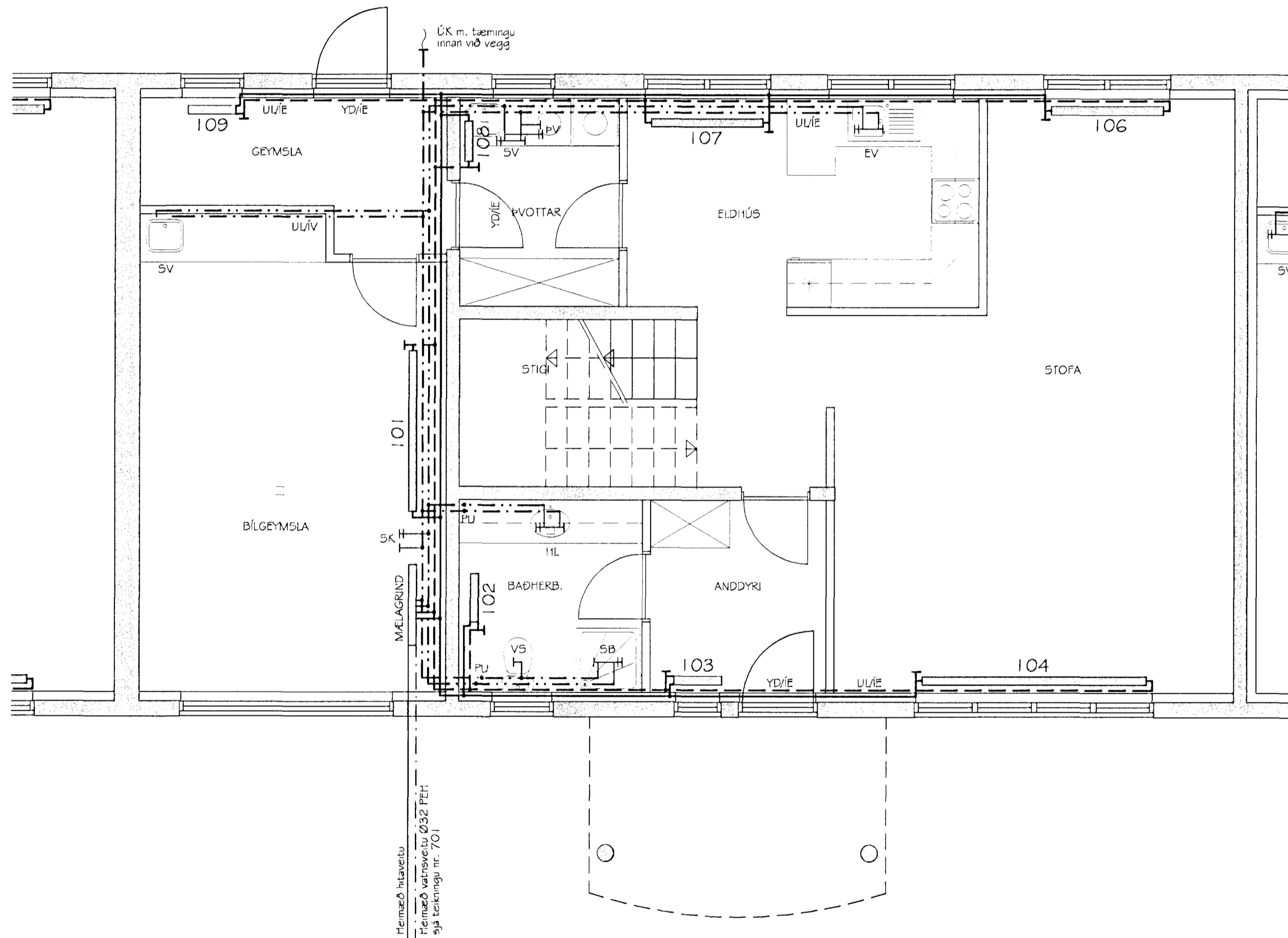
BLÓMVELLIR 31 HITA- OG NEYSLUVATNSLAGNIR GRUNNMYND NEDRI HÆÐAR MKV. 1:50
