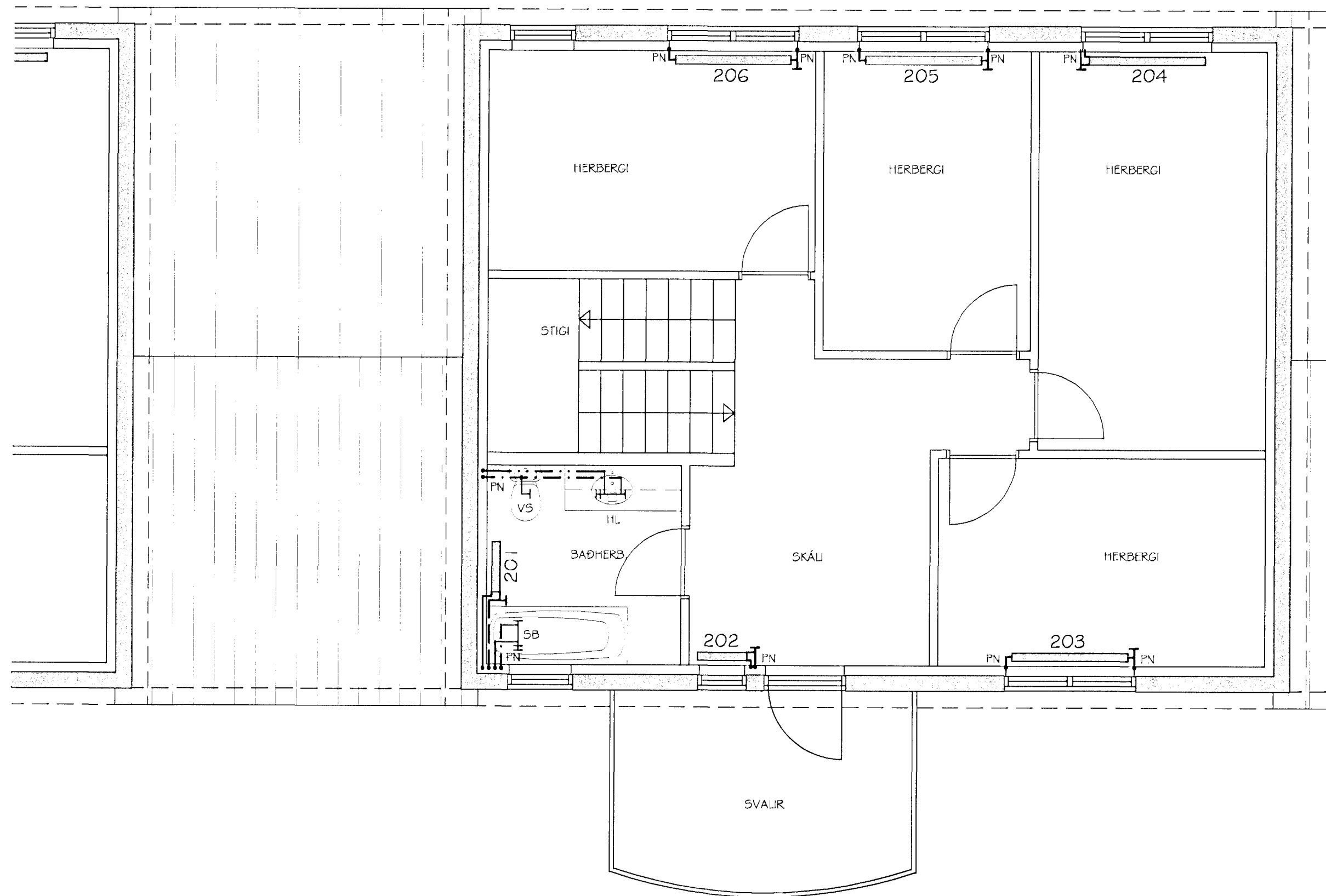
BLÓMVELLIR 3 I HITA- OG NEYSLUVATNSLAGNIR GRUNNMYND NEDRI HÆÐAR MKV. 1:50
