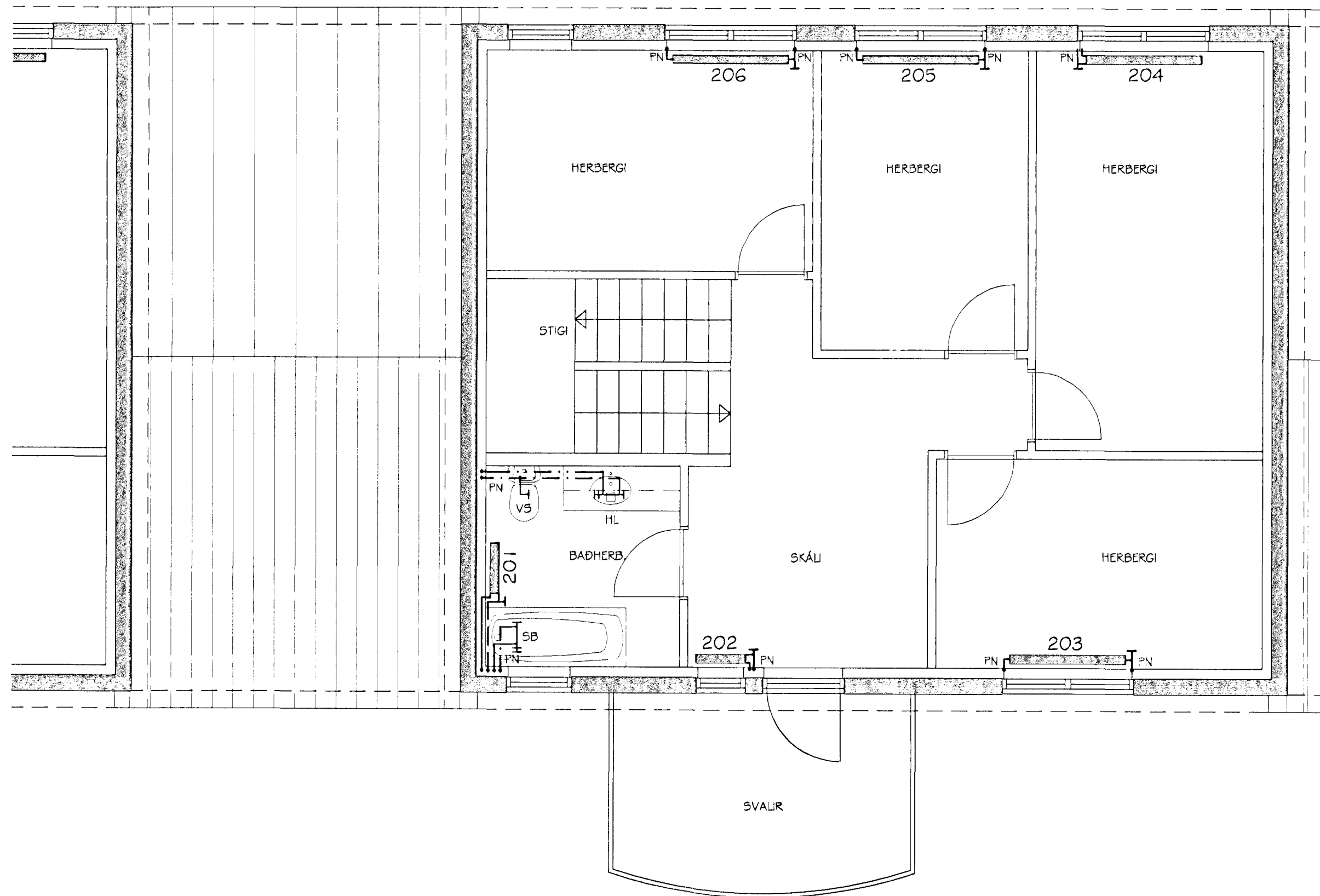
BLÓMVELLIR 33 HITA- OG NEYSLUVATNSLAGNIR GRUNNMYND NEDRI HÆÐAR MKV. 1:50
