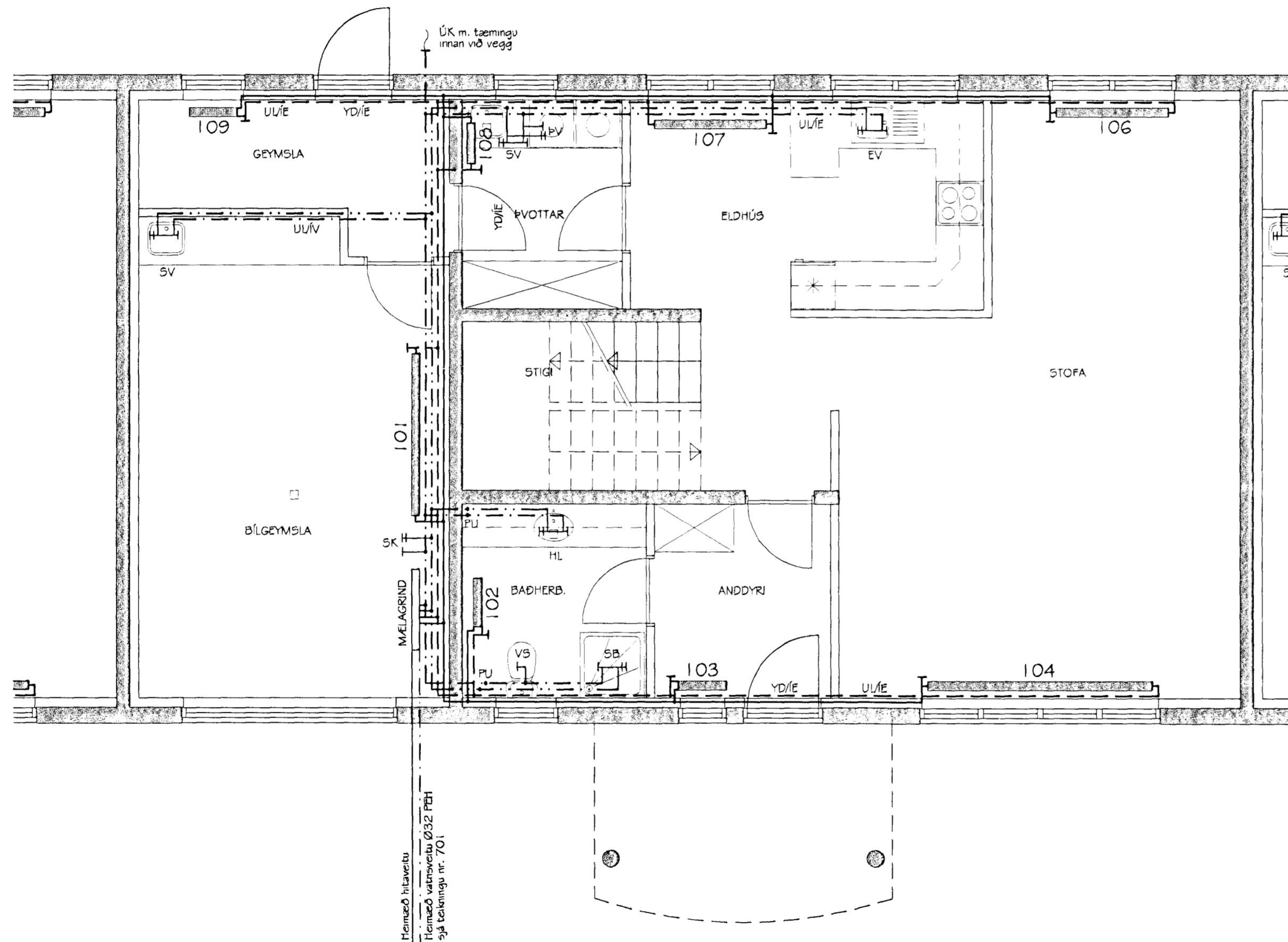
BLÓMVELLIR 33 HITA- OG NEYSLUVATNSLAGNIR GRUNNMYND NEDRI HÆÐAR MKV. 1:50
