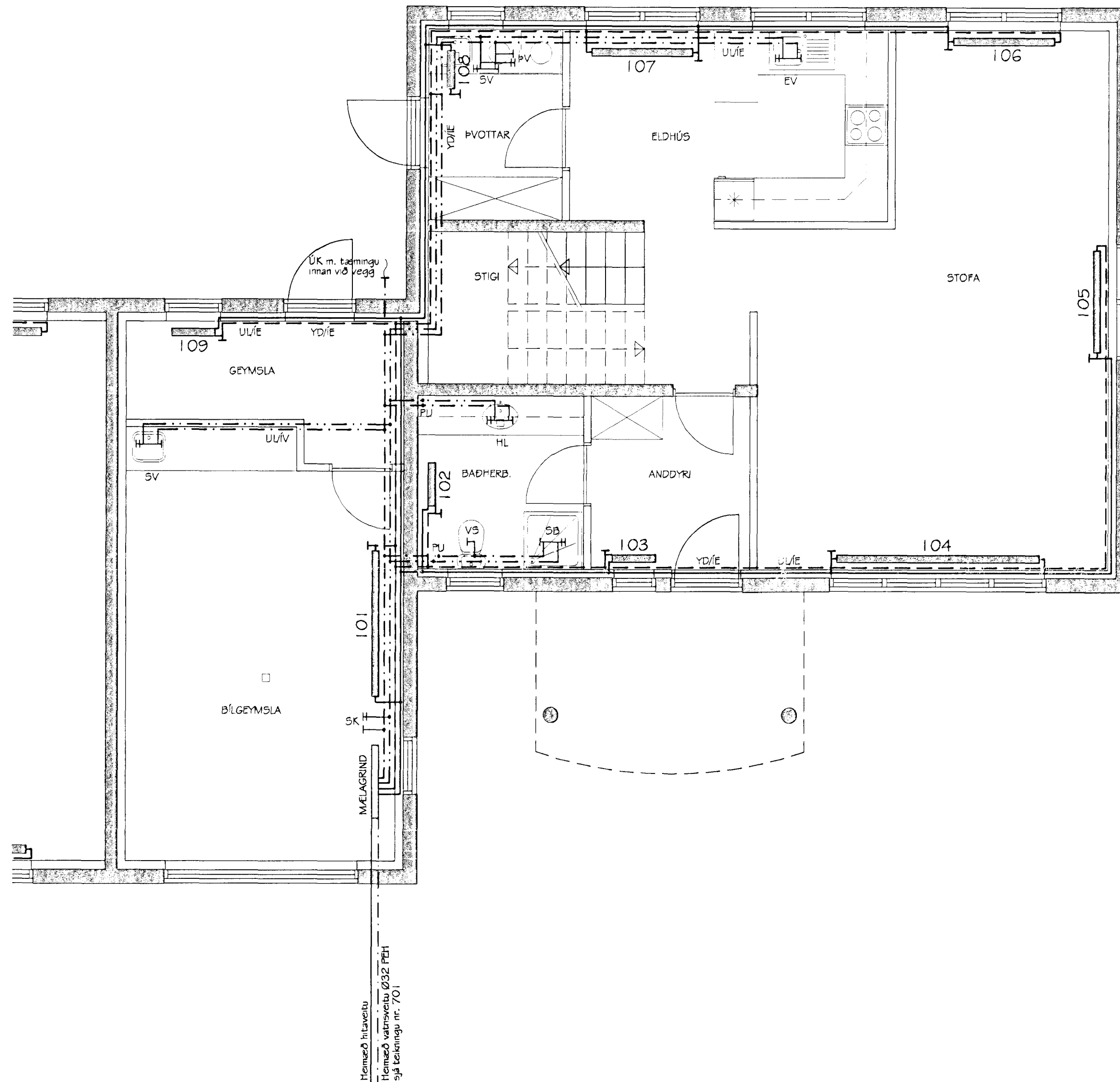
BLÓMVELLIR 35 HITA- OG NEYSLUVATNSLAGNIR GRUNNMYND NEDRI HÆÐAR MKV. 1:50
