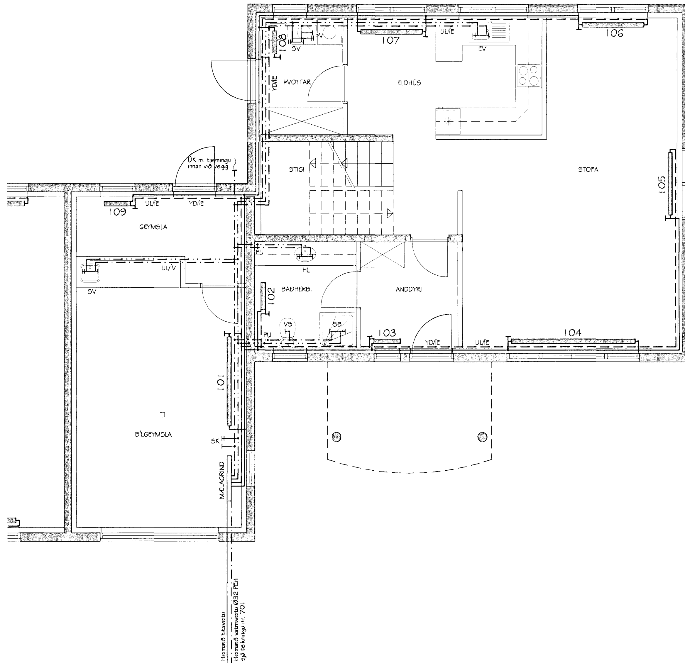
BLÓMVELLIR 35 HITTA- OG NEYSLUVATNSLAGNIR GRUNNMYND NEDRI HÆÐAR MKV. 1:50
