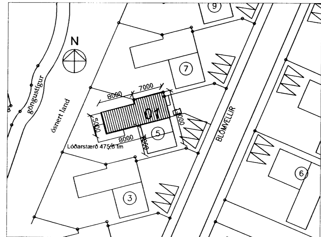
afstöðumynd, 1:500
