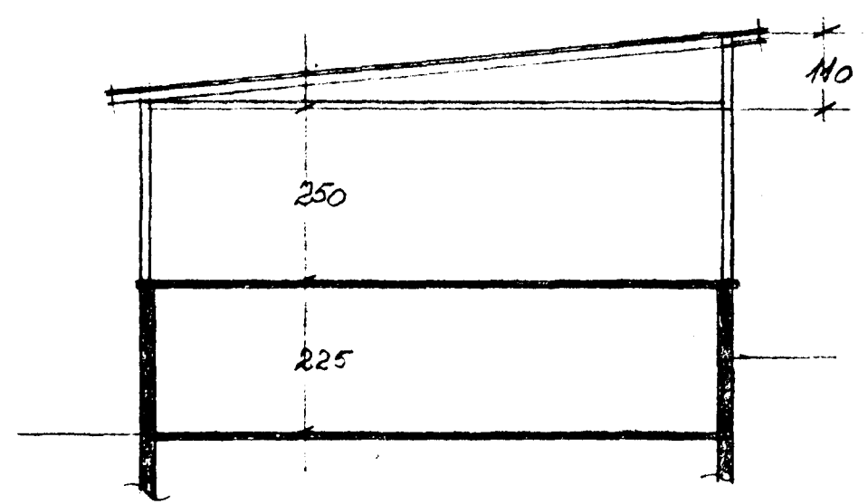
SNID a-a
